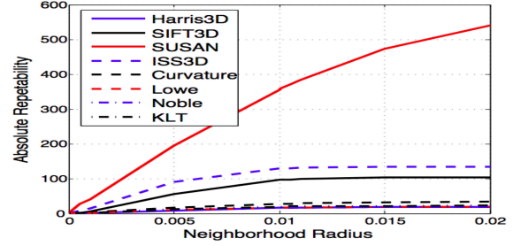
(d) Absolute repeatability for 15^\circ rotation.
