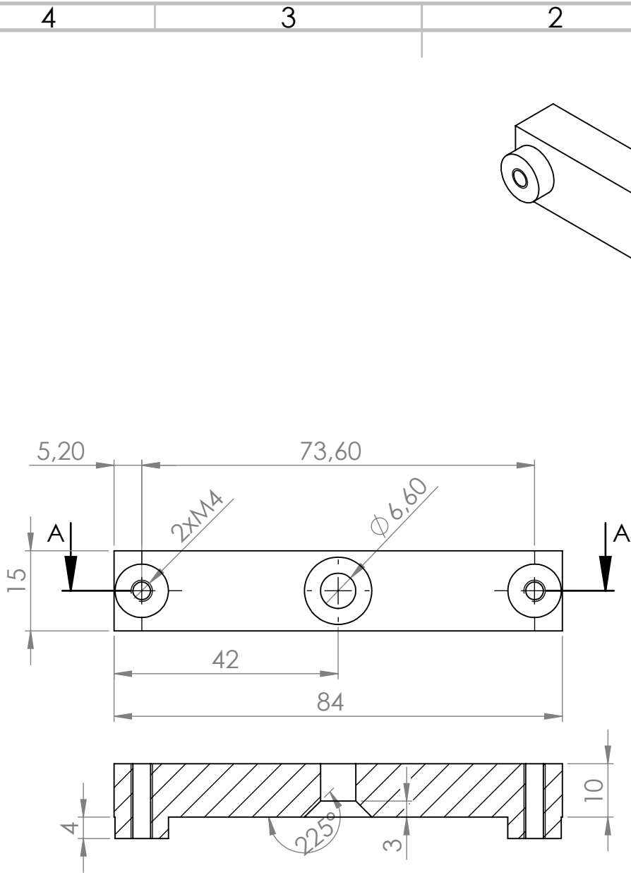
SECTION A-A
