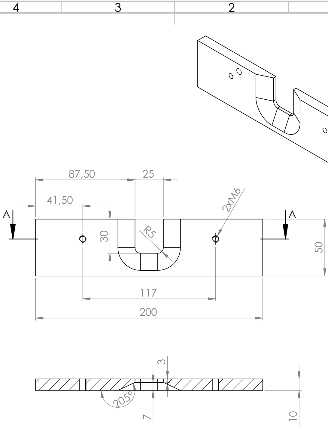
SECTION A-A
