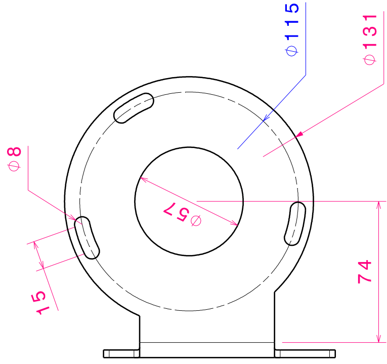
Right view Scale: 1:2
