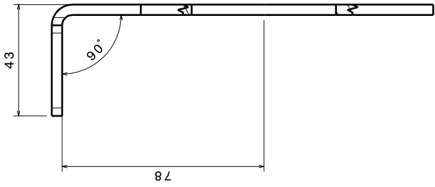
Bottom view Scale: 1:1
