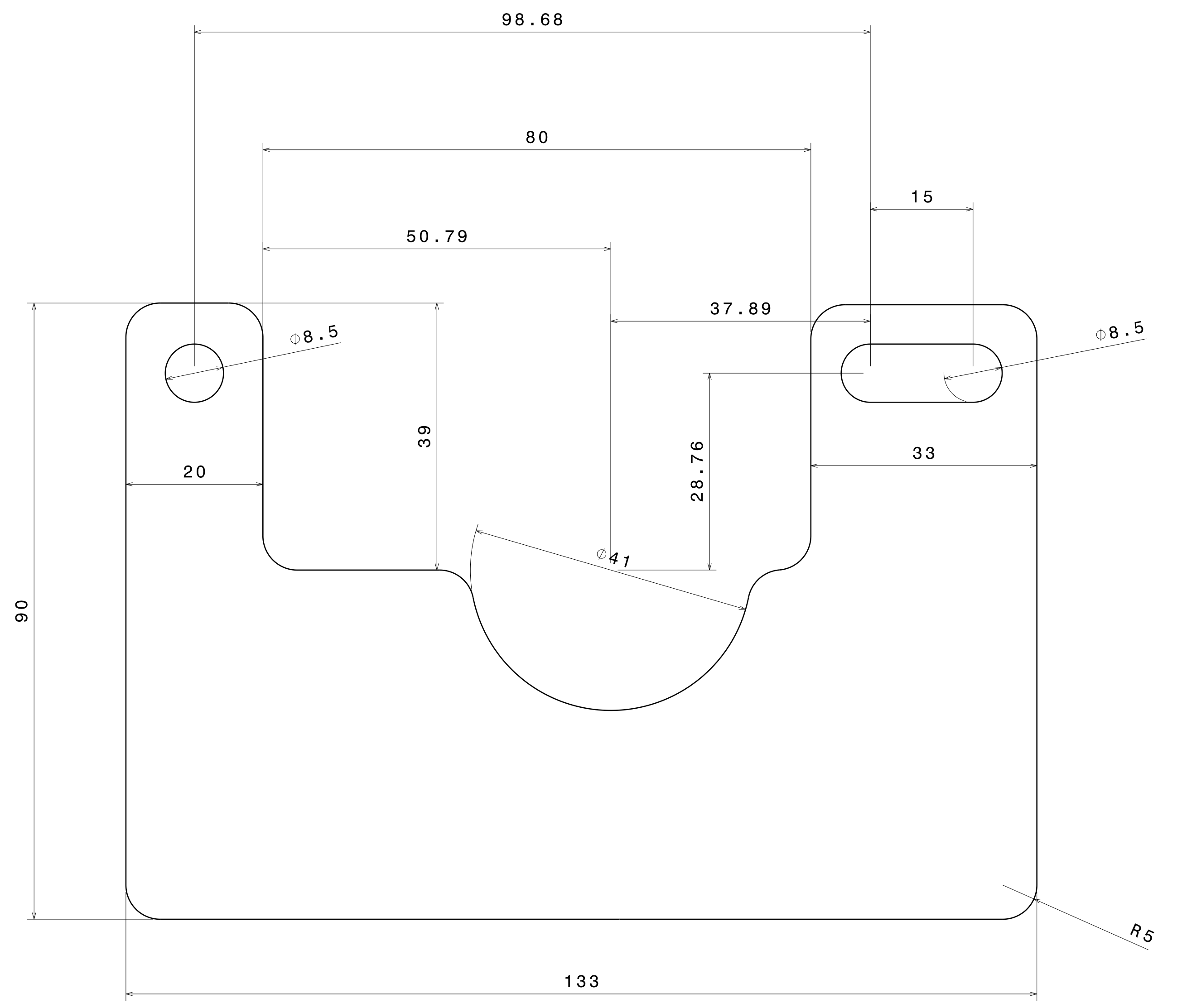
Right view Scale: 2:1
