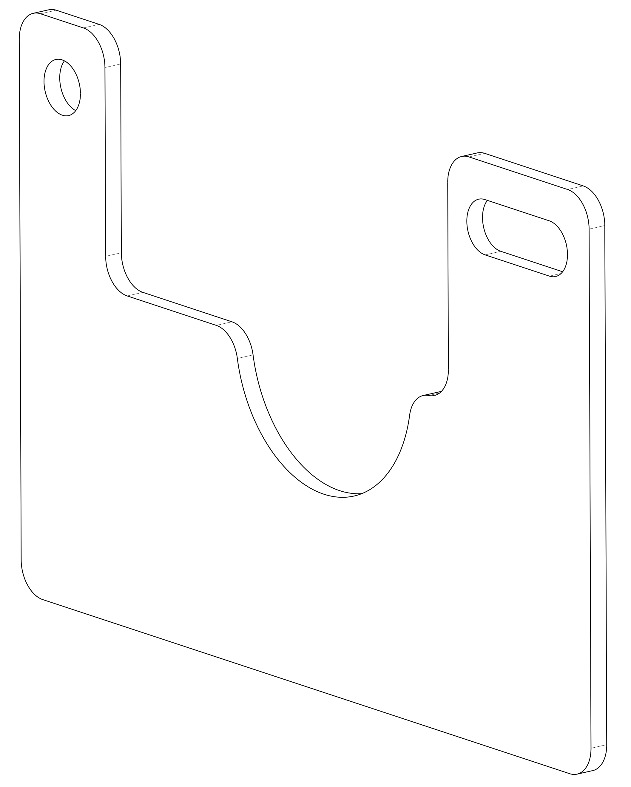
Isometric view Scale: 3:1
