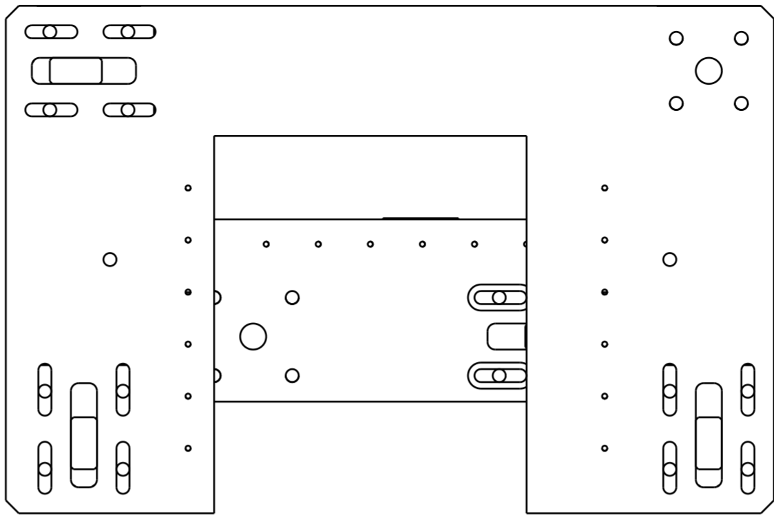
Bottom view Scale: 1:2
