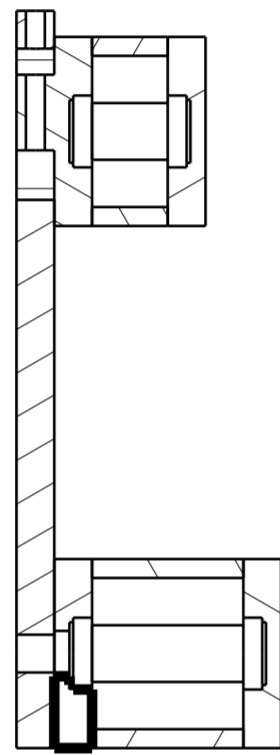
Section view A-A Scale: 1:2
