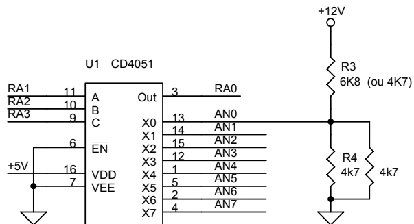
Multiplexer Analógico
