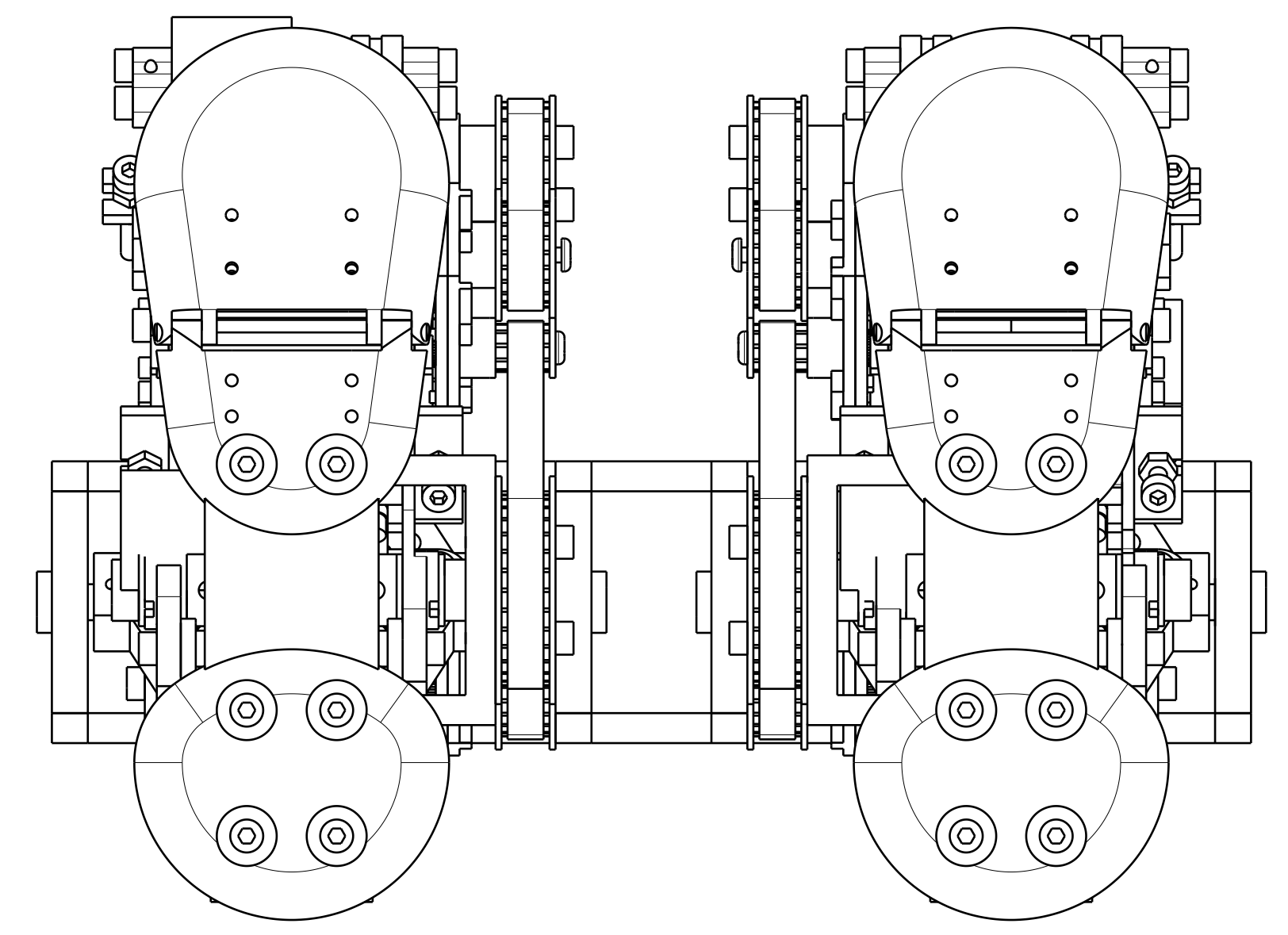
Rear view Scale: 1:1
