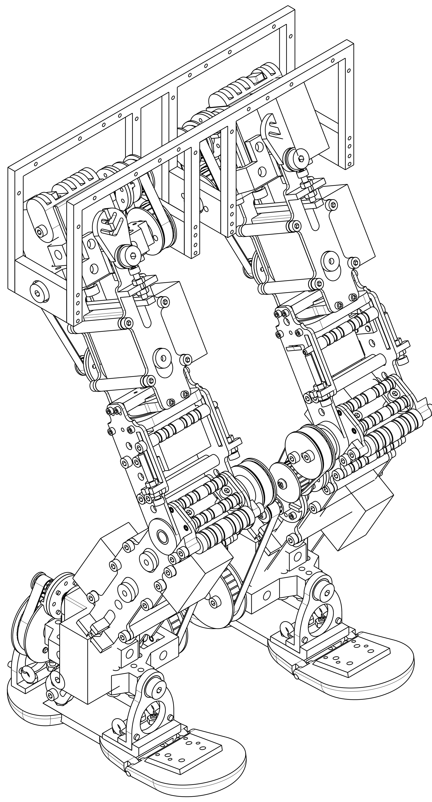
Isometric view Scale: 1:1
