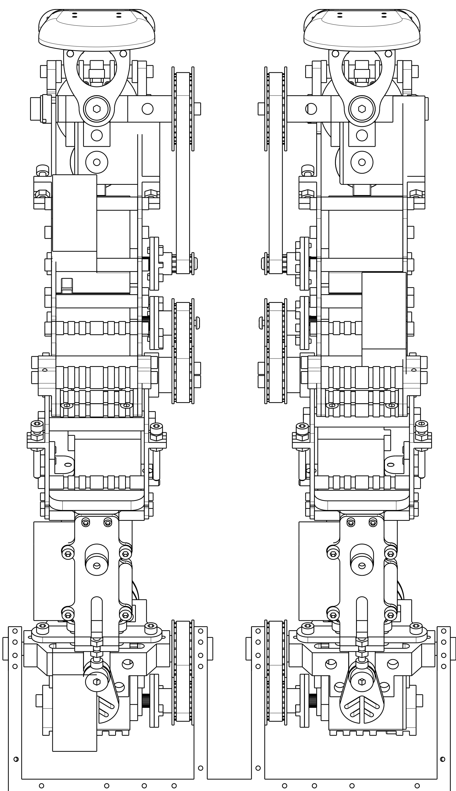
Top view Scale: 1:1
