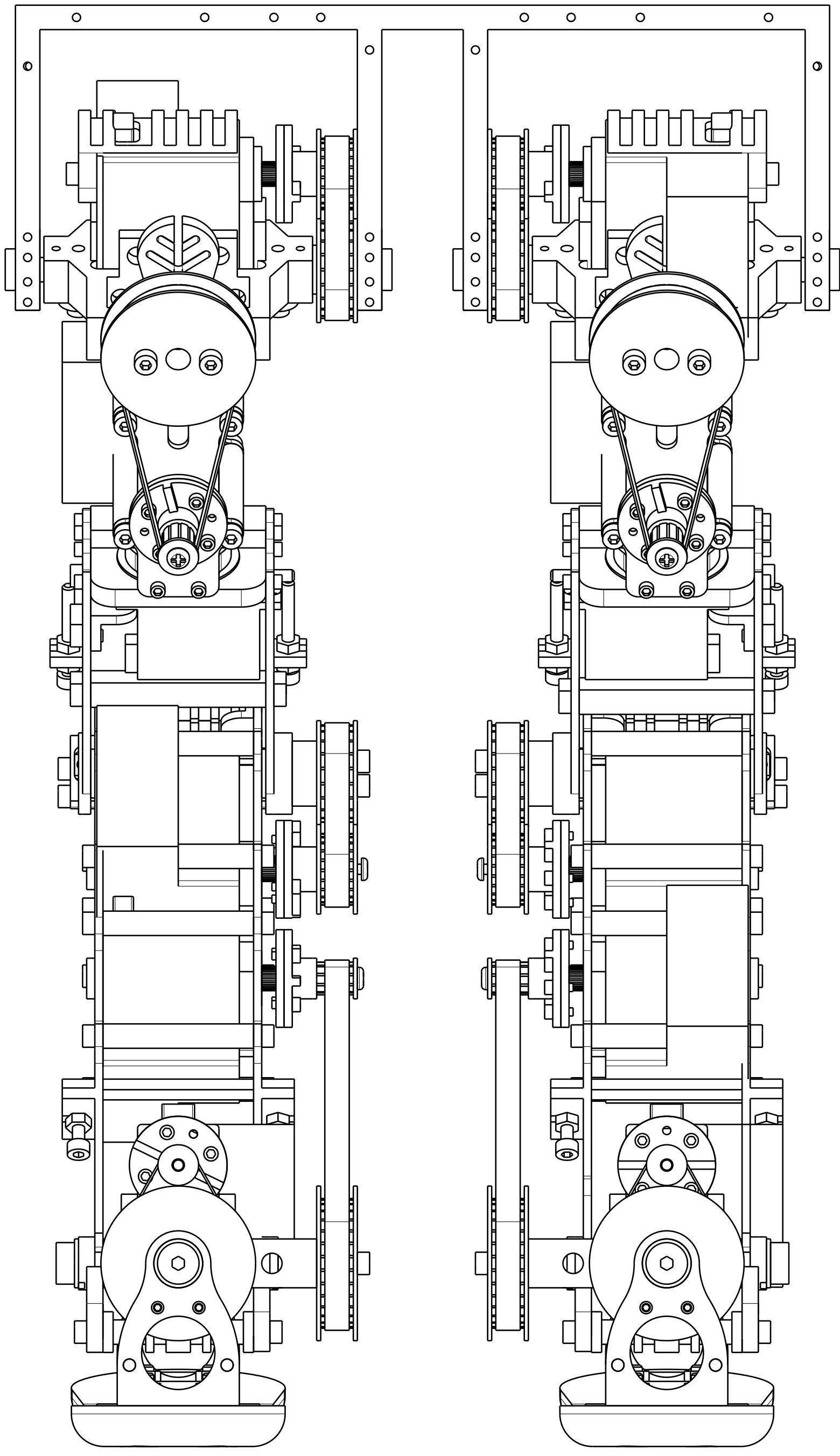
Bottom view Scale: 1:1
