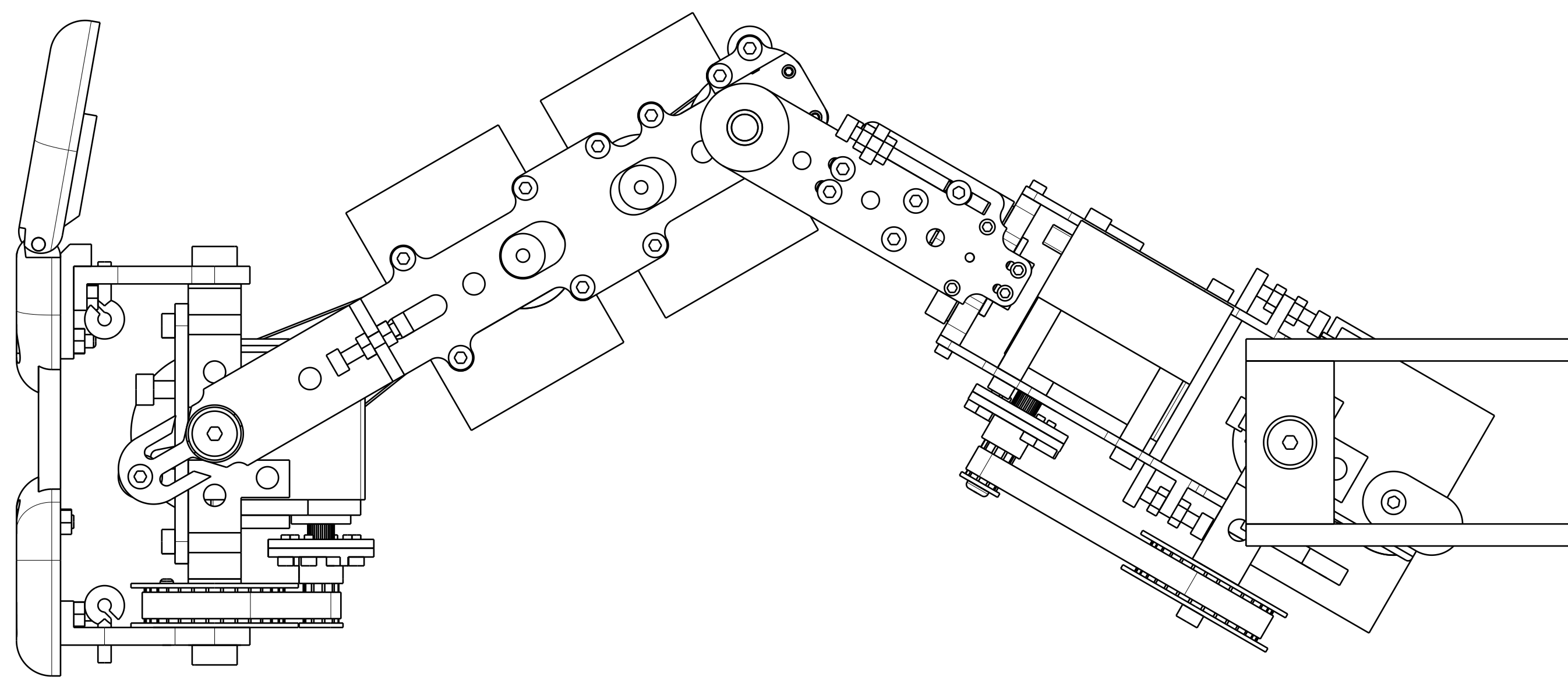
Left view Scale: 1:1
