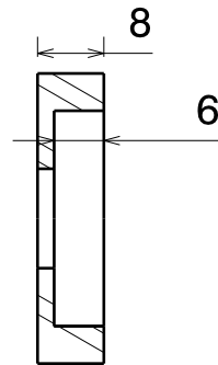
Section view A-A Scale: 1:1
