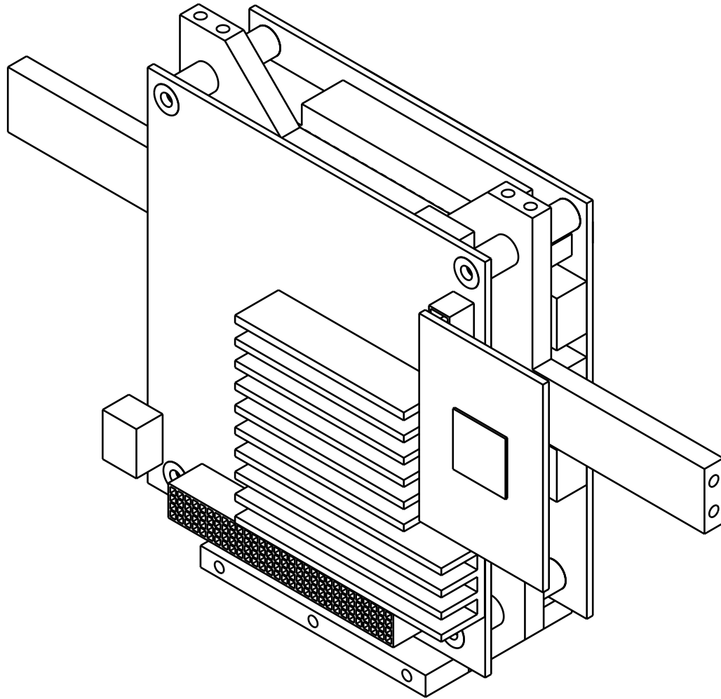
Isometric view Scale: 1:1
