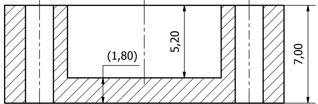
A-A ( 6 : 1 )
