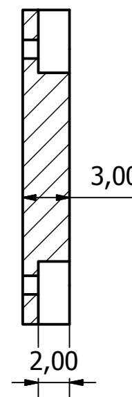
A-A ( 3 : 1 )
