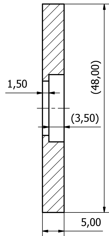
B-B ( 2 : 1 )
