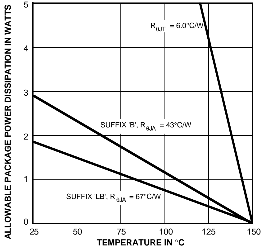
Dwg. GP-049-2
