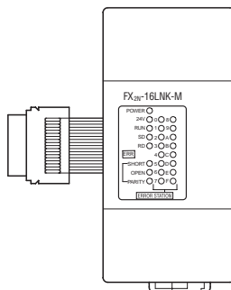
FX2N-16LNK-M
