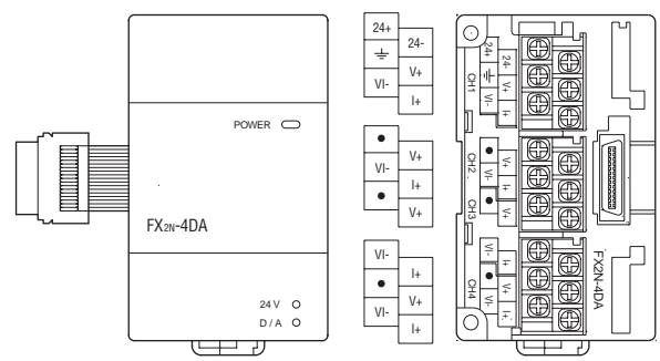
FX2N-4DA
