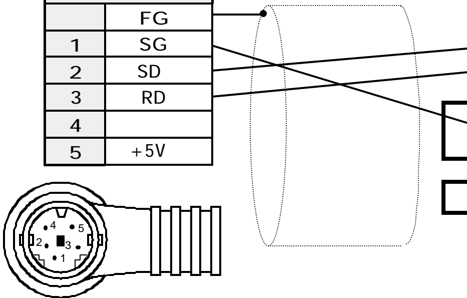
5 Pin Mini Din Source One Molding connector
