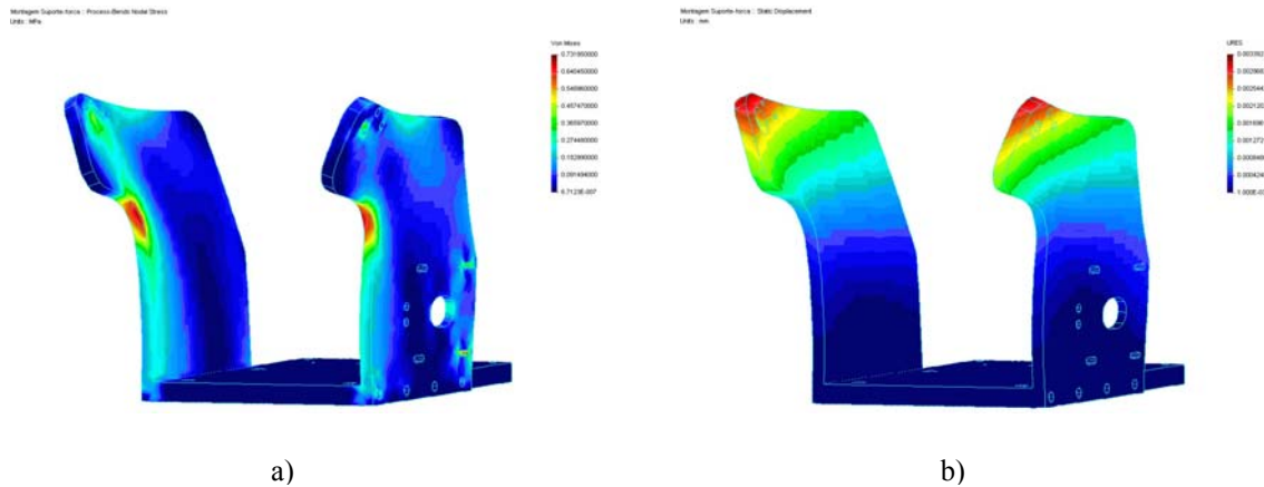
Fig. 5 – Análise estática da estrutura , a) tensões máximas , b) deslocamentos máximos.
