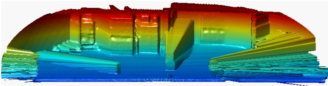
Fig. 34 – Resultado obtidos a uma velocidade angular do laser de 21,1°/s.
