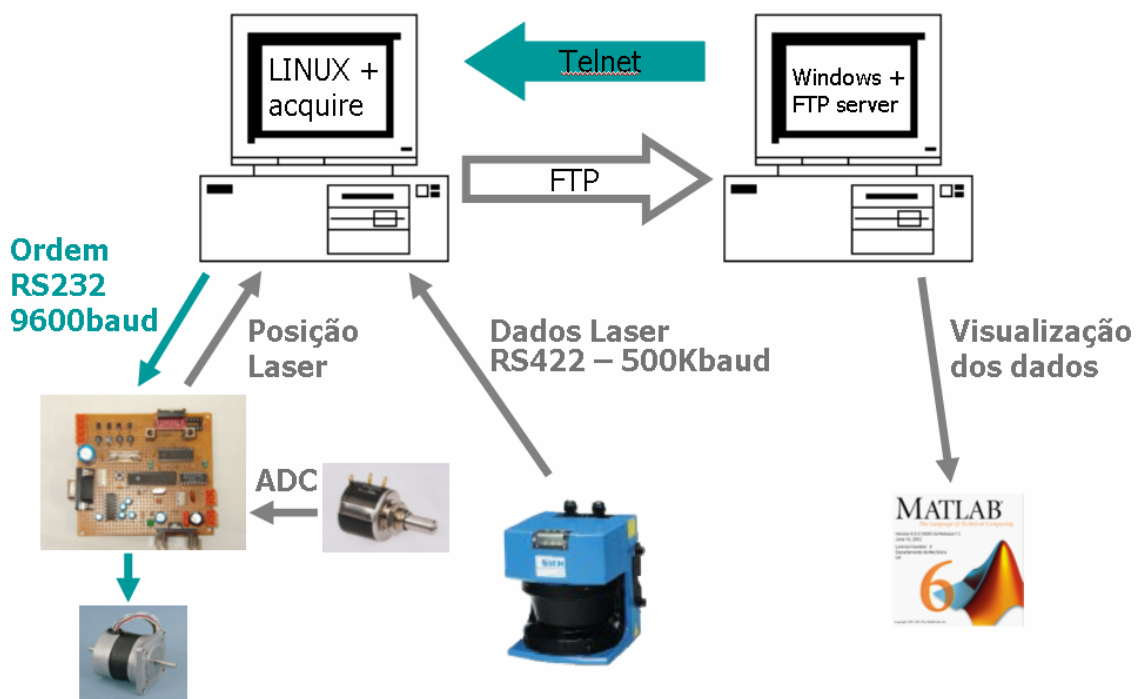
Fig. 32 – Diagrama da aquisição de dados.
