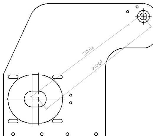
Fig. 6 – Distâncias dos entre-eixos.
