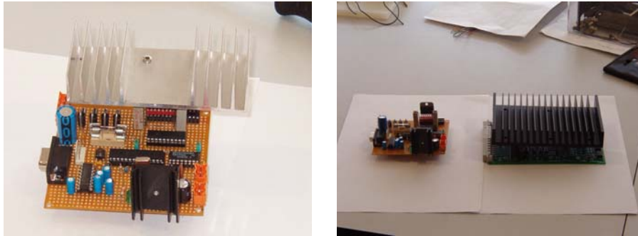
Fig. 12 – Aspecto final da placa de controlo e comparação de tamanho com carta de potência na solução inicial.
