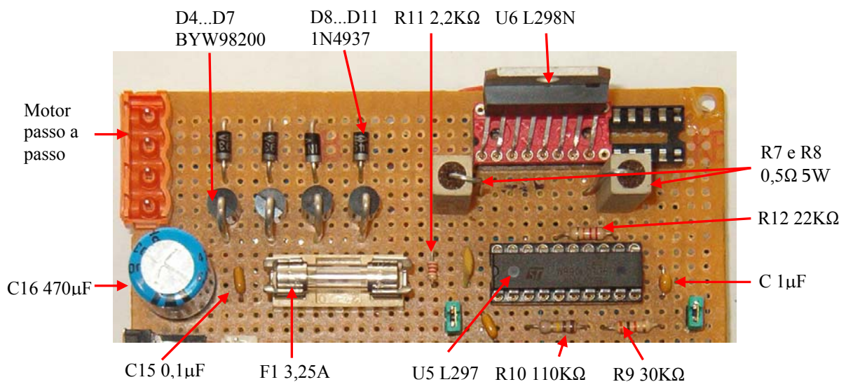
Fig. 17 – Identificação dos vários componentes – Gerador de Pulsos e Circuito de Potência.
