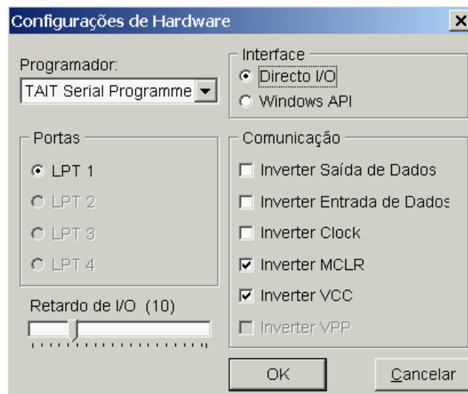
Fig. 22 – Configuração do IC-Prog [22] (hardware - continuação).
