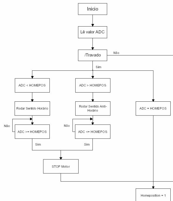
Fig. 31 – Diagrama de blocos da inicialização da placa controladora.
