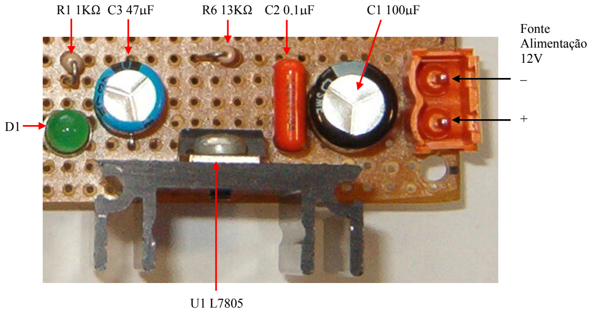
Fig. 14 – Identificação dos vários componentes – Fonte de Alimentação.
