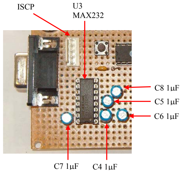
Fig. 16 – Identificação dos vários componentes – Comunicação RS232.
