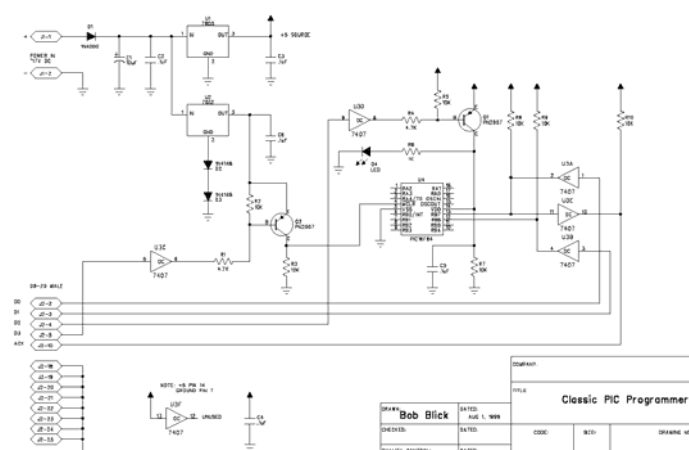
Fig. 18 – Circuito electrónico do programador de PIC's.
