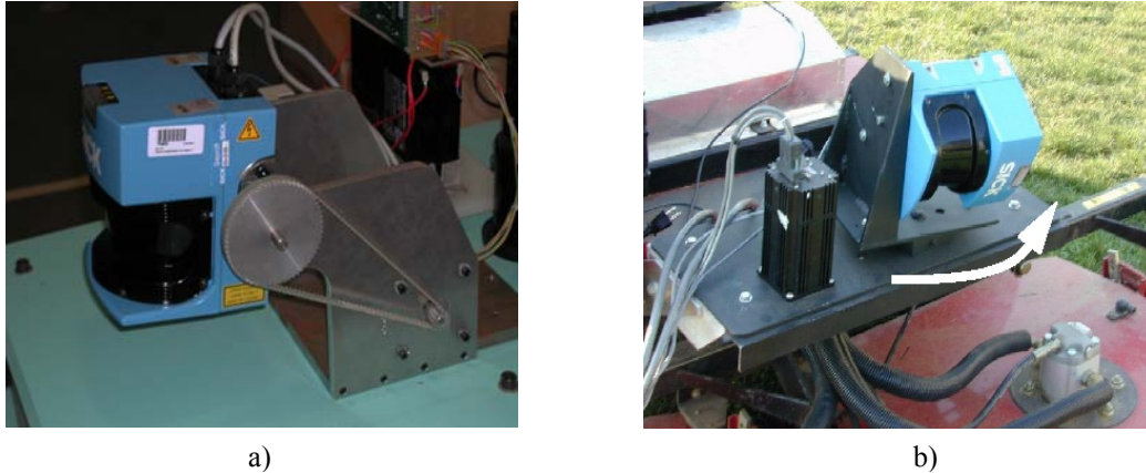
Fig. 2 – Forma de “varrimento” do laser, a) na horizontal, b) na vertical [7].
