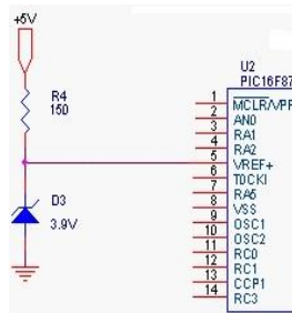
Fig. 28 – Circuito Vref+.
