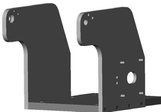
Fig. 4 – Estrutura mecânica final de suporte do laser.
