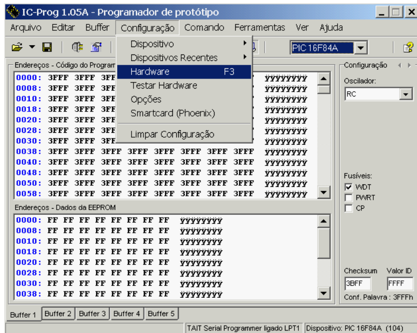
Fig. 21 – Configuração do IC-Prog [22] (hardware).
