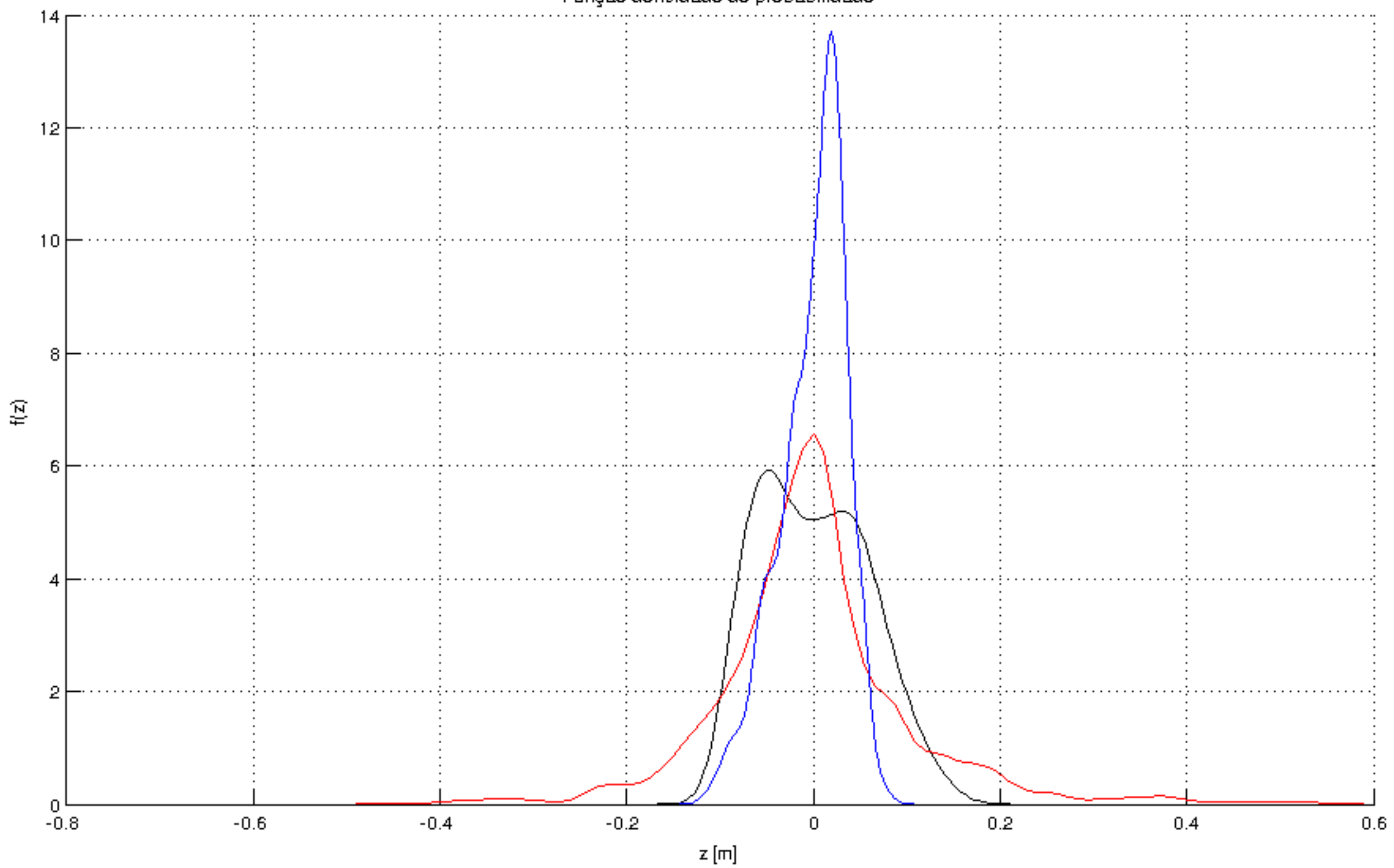
Função densidade de probabilidade
