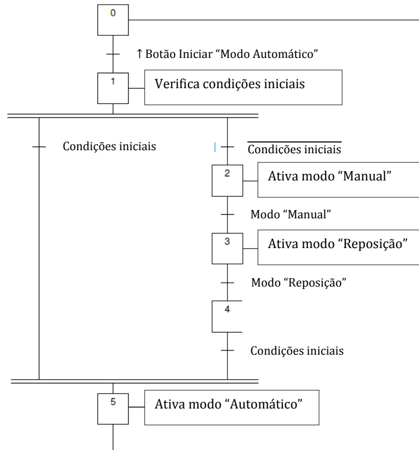
Figura 22 - Grafcet de colocação da estação em "modo automático".
