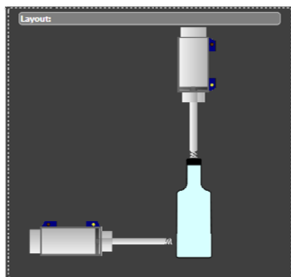
Figura 63 – “Layout” (ecrã de monitorização e controlo da estação 1) - (Avanço do cilindro 2).
