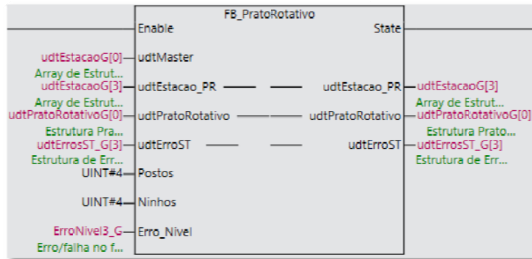
Figura 37 - Function Block de controlo do prato rotativo.
