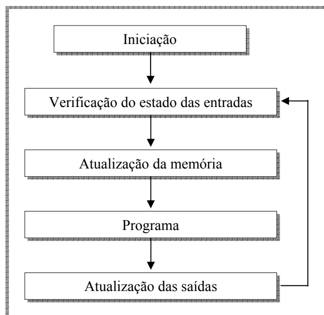
Figura 7 - Ciclo de processamento de um PLC.
