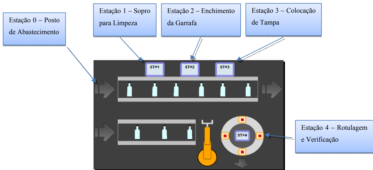
Figura 45 - Layout do Caso de Estudo 1.
