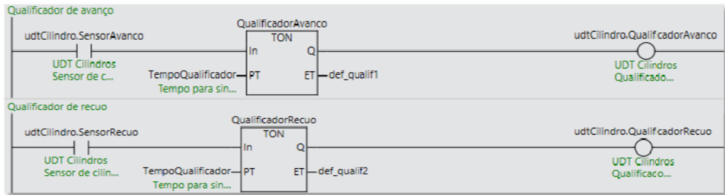
Figura 31 – Implementação do timer para detecção dos erros de “TimeOut” (linguagem Ladder).
