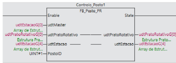
Figura 38 - Function Block de controlo dos postos de trabalho.
