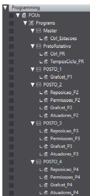
Figura 76 - Árvore de navegação dos POU's do caso de estudo 2.
