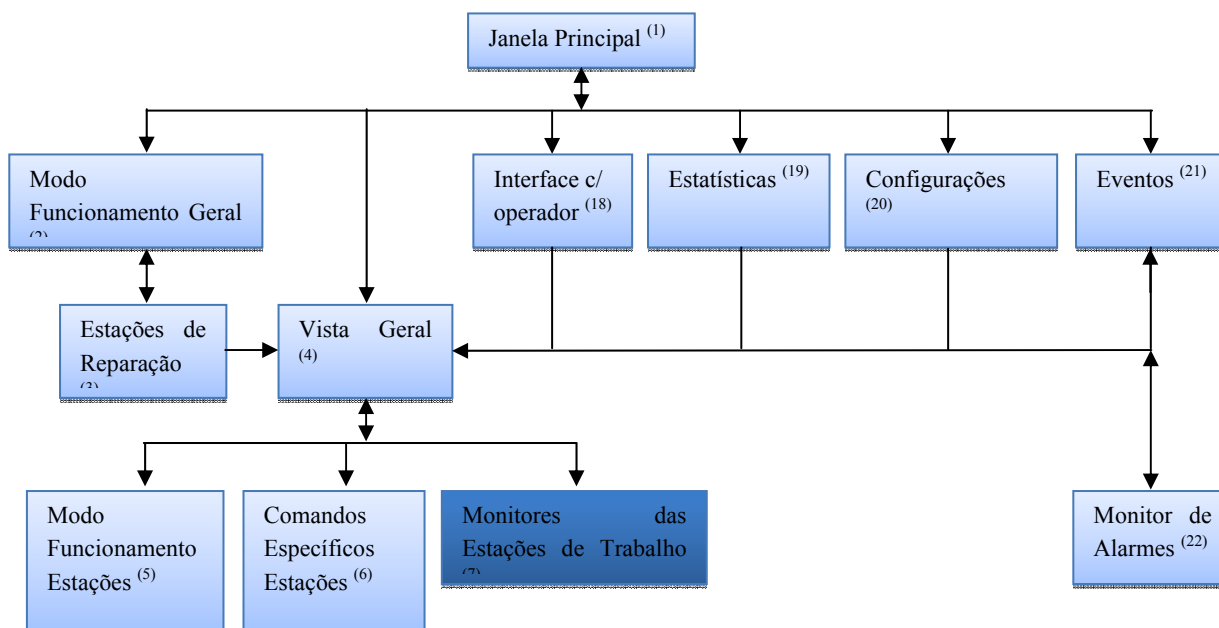
Figura 47 - Estrutura de ecrãs da consola do caso de estudo 1.
