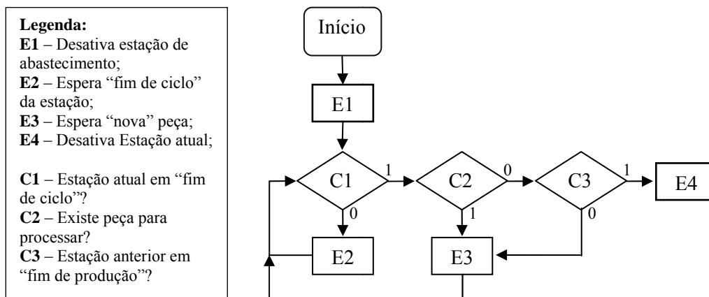
Figura 24 - Fluxograma do processo de colocação de "fim de produção" da estação.
