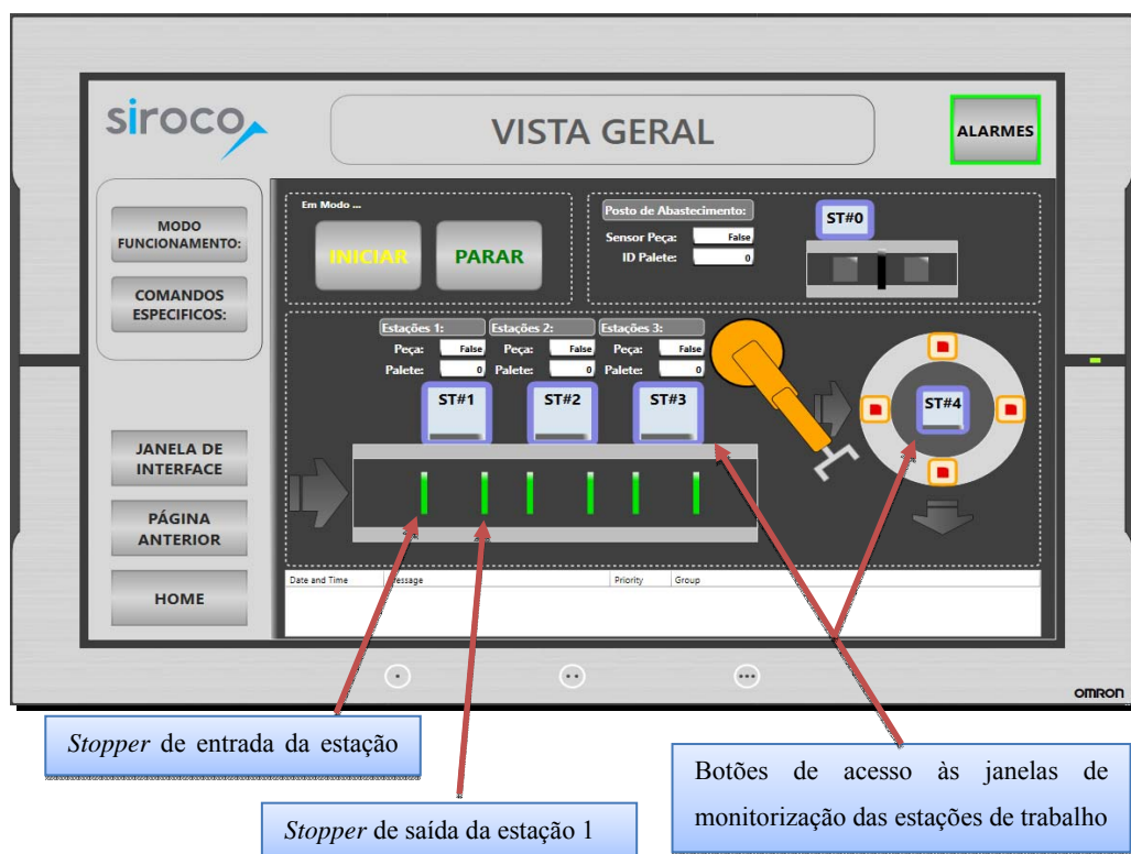
Figura 57 - Ecrã "Vista Geral" – Caso de Estudo 1.
