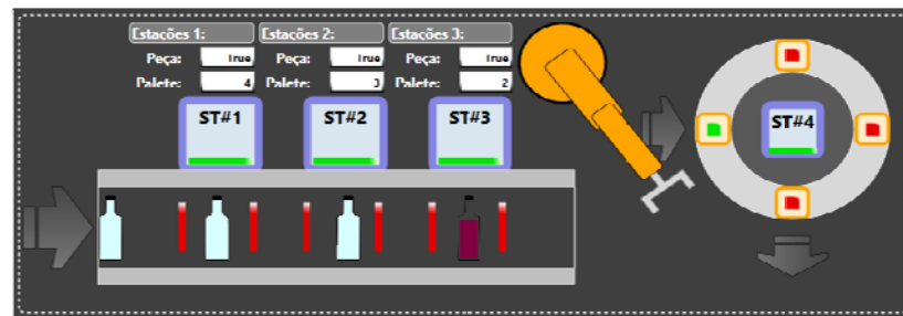
Figura 69 - "Layout" (ecrã "Vista Geral") - início de ciclo do prato rotativo.
