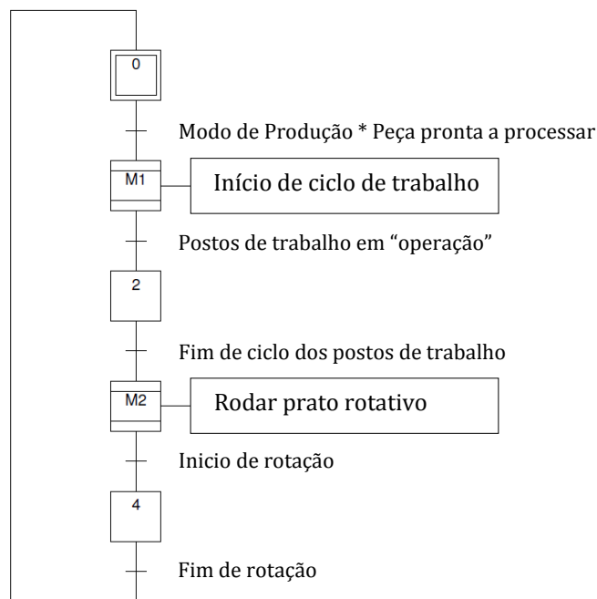
Figura 34 - Grafcet de controlo e gestão do prato rotativo em modo automático.
