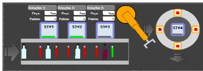
Figura 68 - "Layout" (ecrã "Vista Geral") - garrafa da paleta 3 rumo ao prato rotativo.
