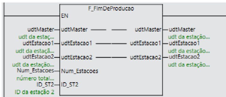
Figura 21 – Function de controlo do "fim de produção" das estações.
