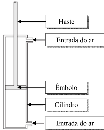
Figura 29 - Cilindro pneumático (duplo efeito) [4].
