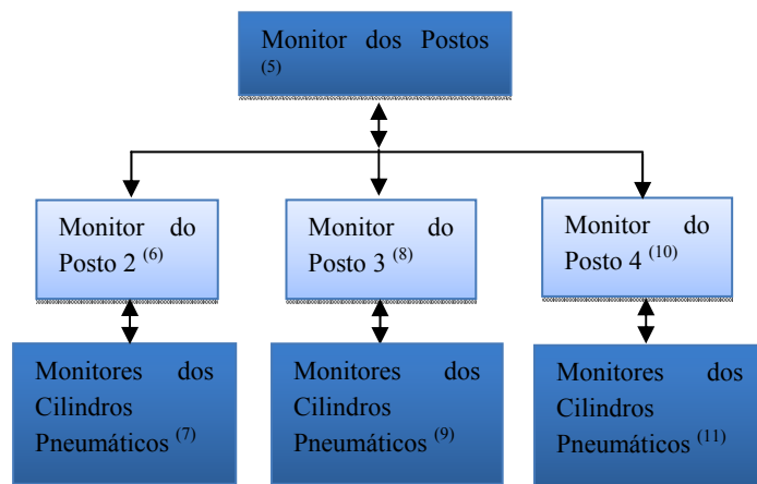
Figura 78 - Estrutura de ecrãs do grupo "Monitor dos Postos de Trabalho".
