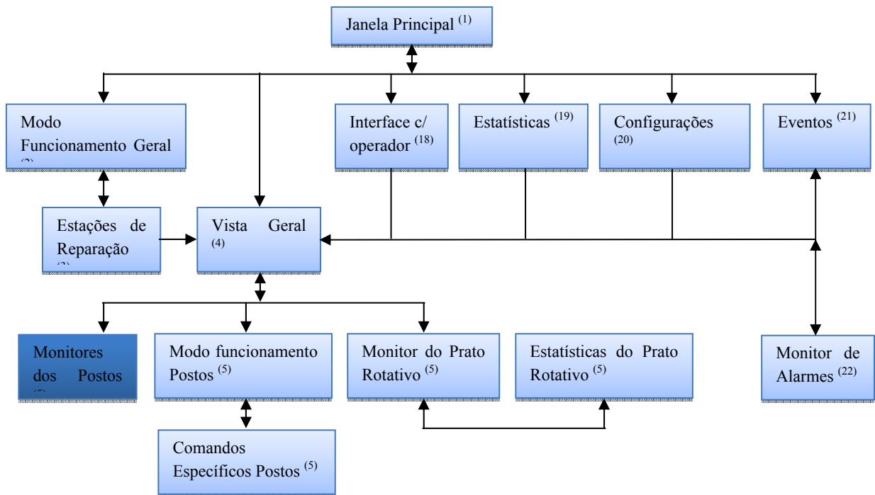
Figura 77 - Estrutura de ecrãs da consola do caso de estudo 2.
