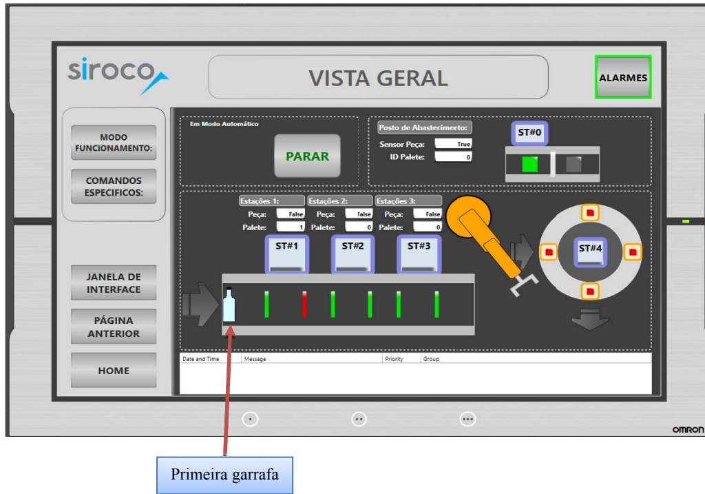
Figura 58 - Ecrã "Vista Geral" - entrada da primeira garrafa.
