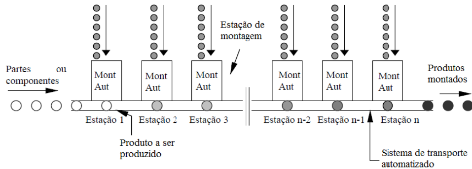
Figura 2 - Configuração geral de sistemas de montagem automatizados [4].
