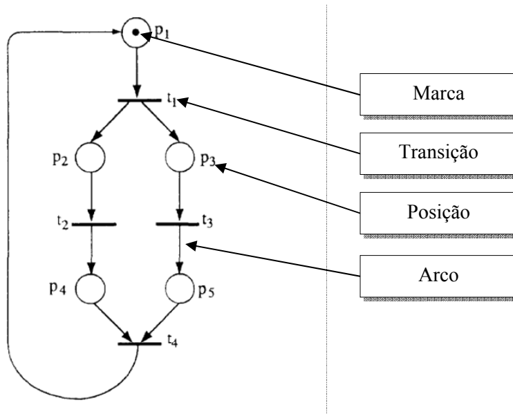
Figura 11 – Exemplo de representação gráfica de uma Petri Net [22].
