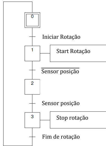
Figura 36 - Grafcet de controlo e gestão da rotação do prato.
