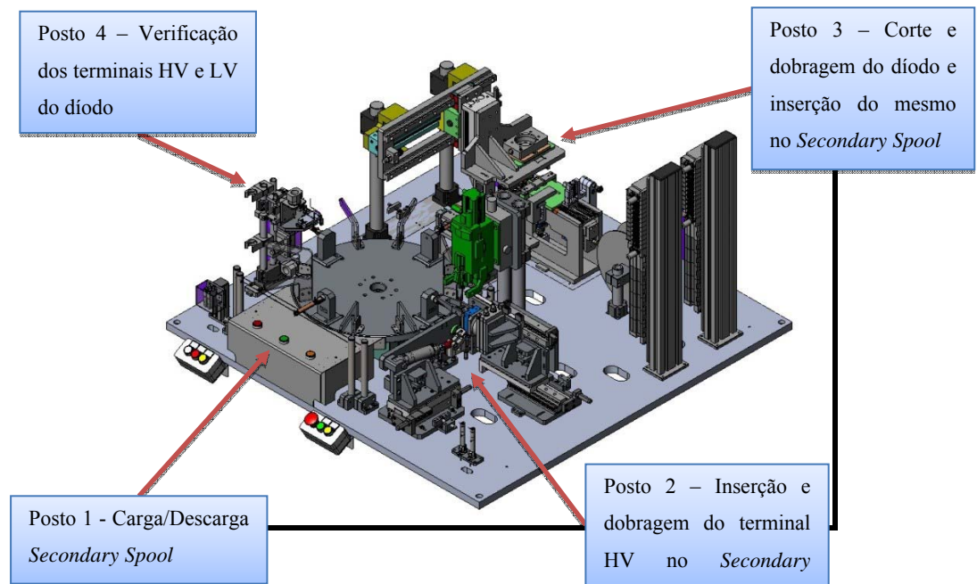
Figura 75 - Layout do Caso de Estudo 2.
