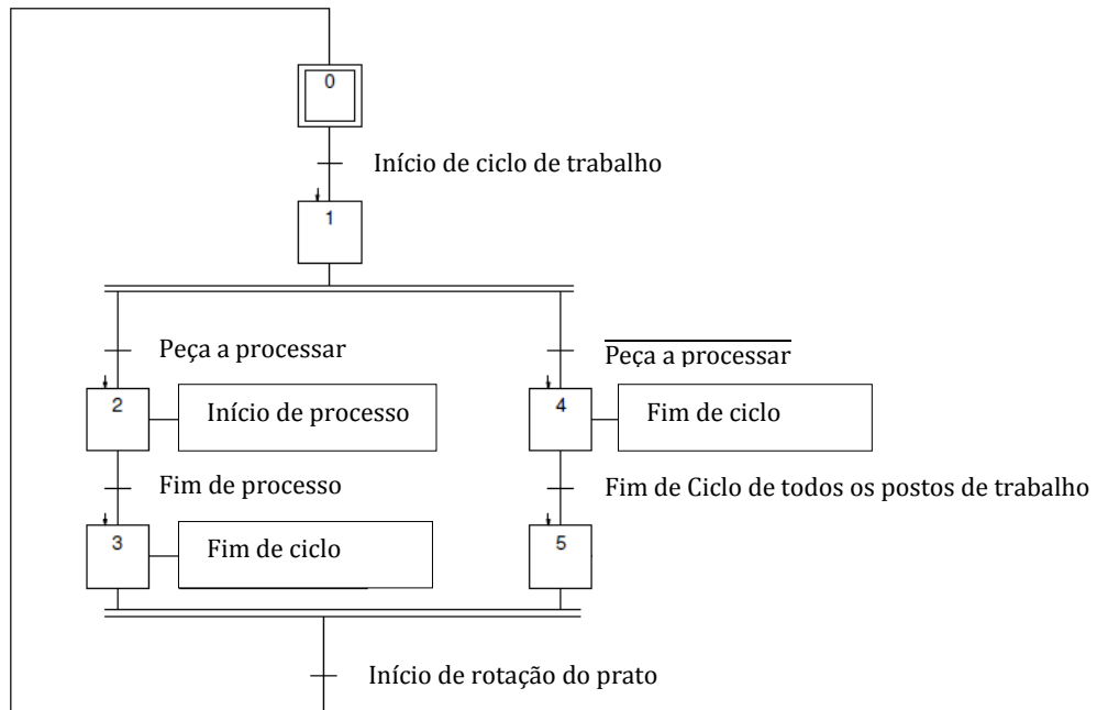
Figura 35 - Grafcet de controlo e gestão do posto de trabalho.
