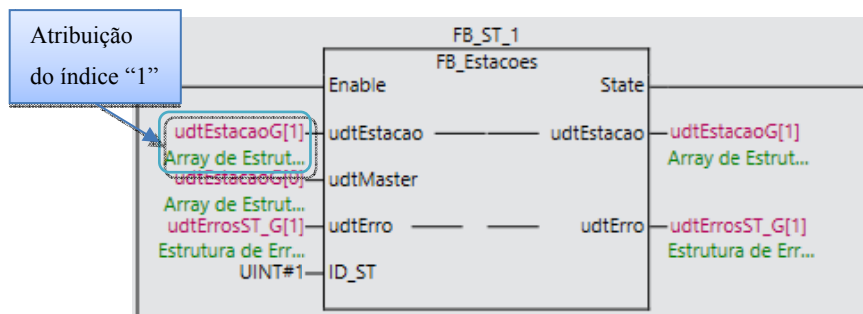
Figura 27 - Function Block de controlo da estação de trabalho 1.
