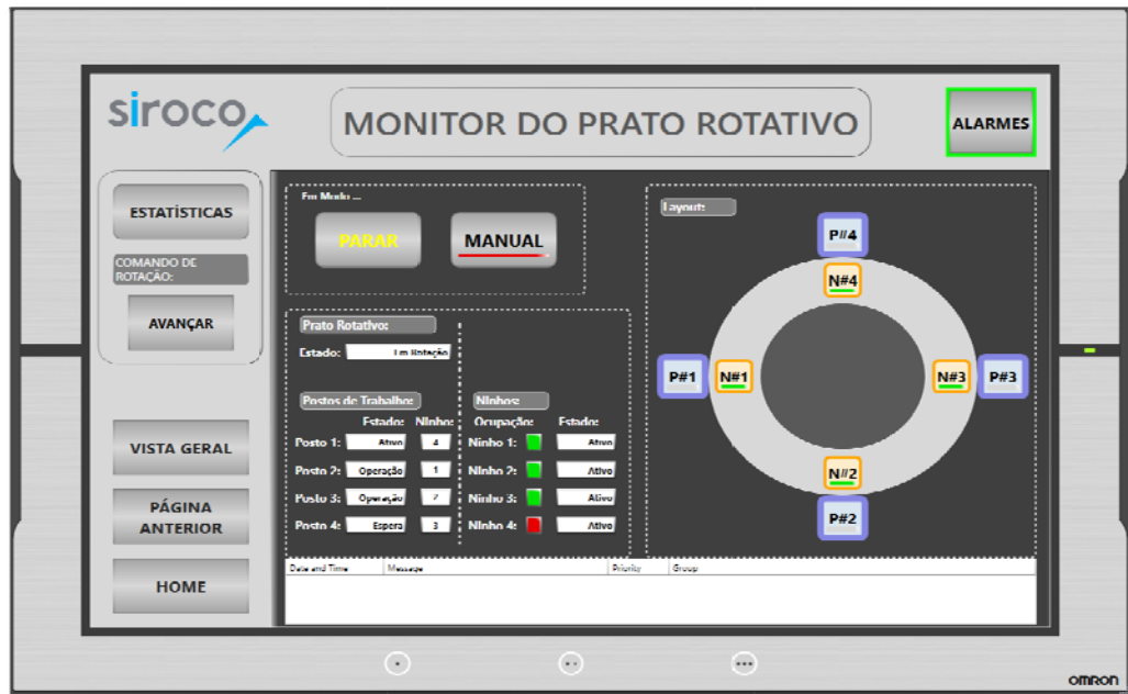
Figura 83 - Ecrã "Monitor Prato Rotativo", Postos 2 e 3 em operação.
