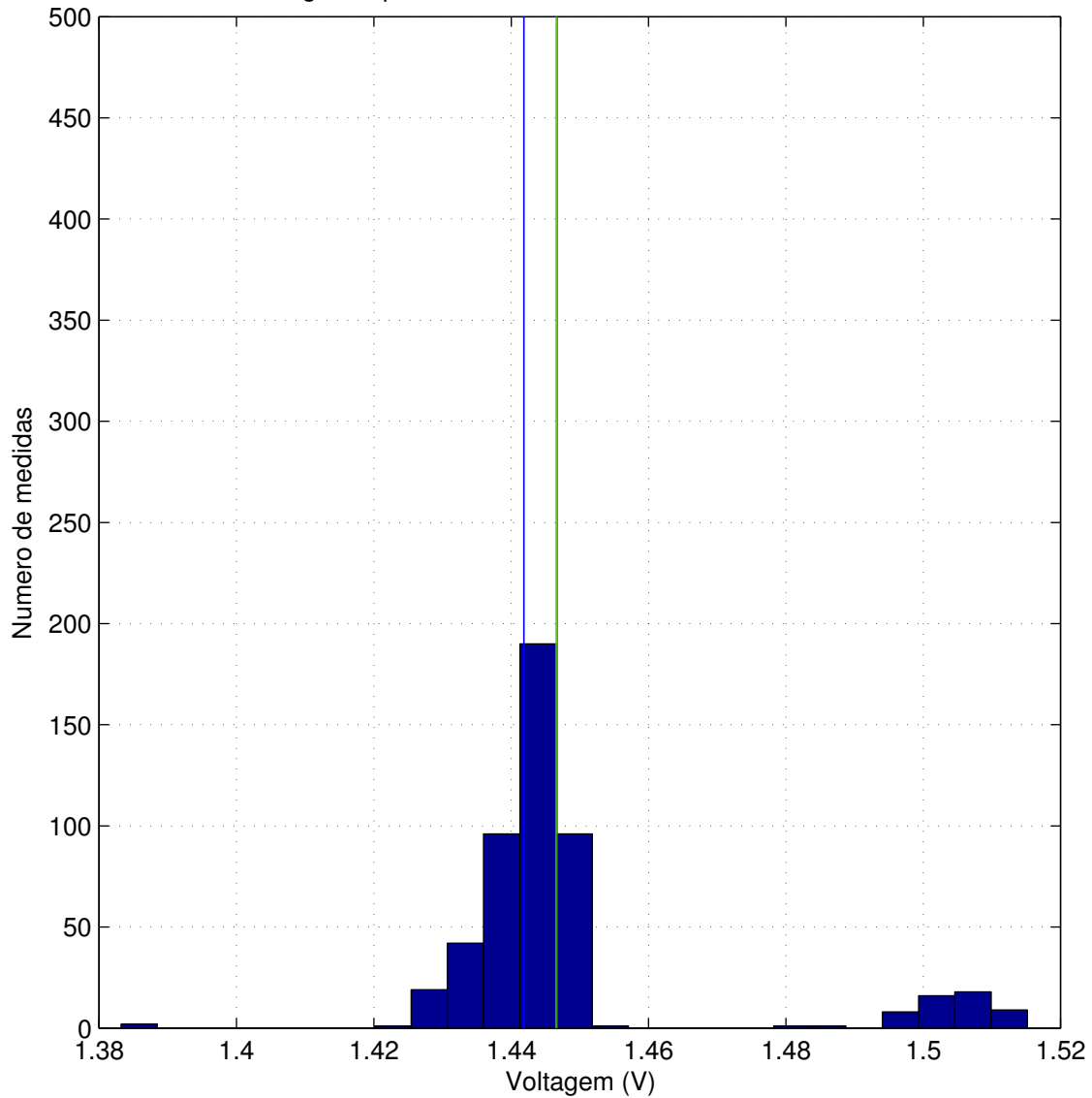
Histograma para 20 cm leituras de 1 em 1 cm com FANUC
