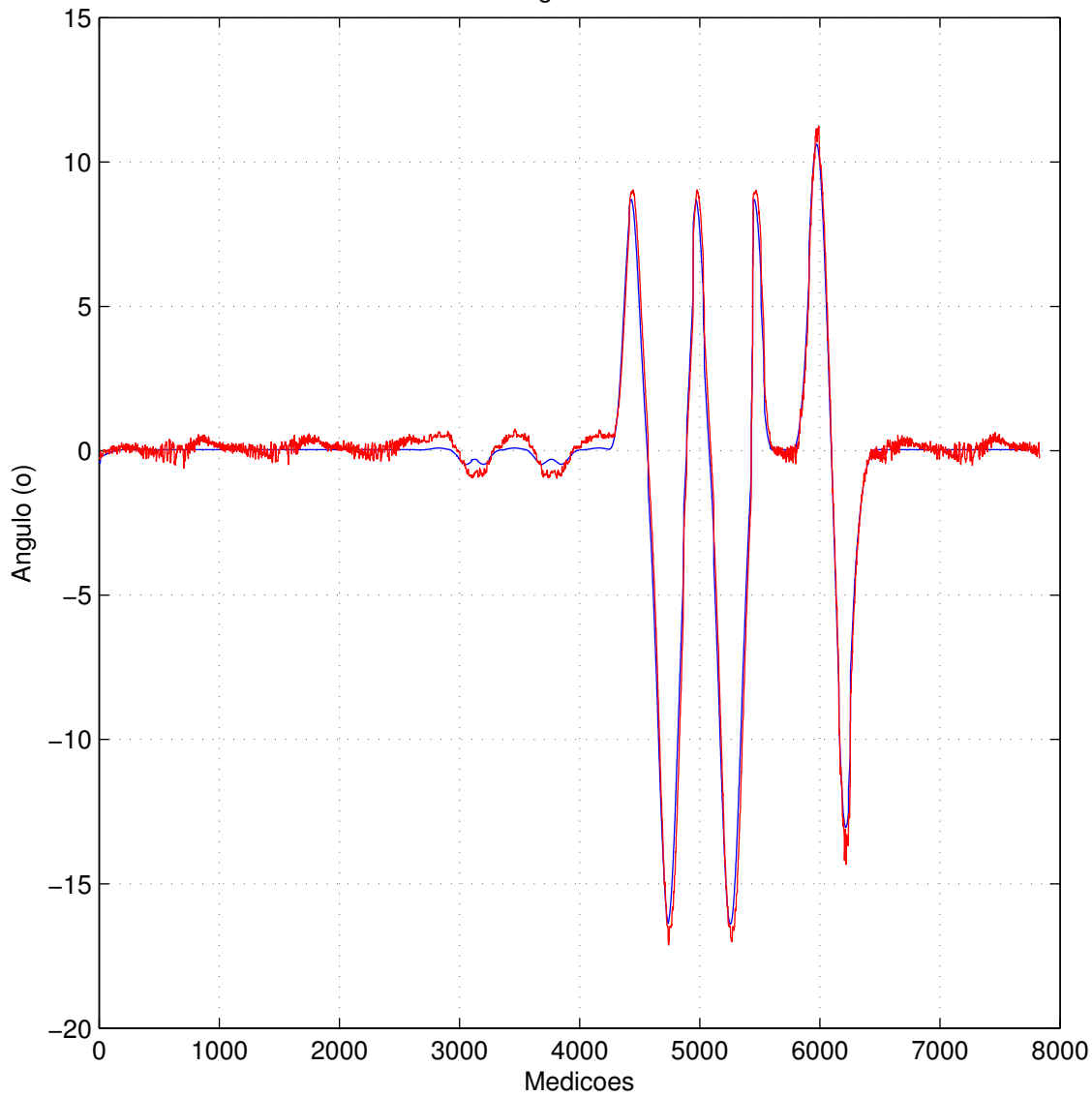
Angulo Pitch
