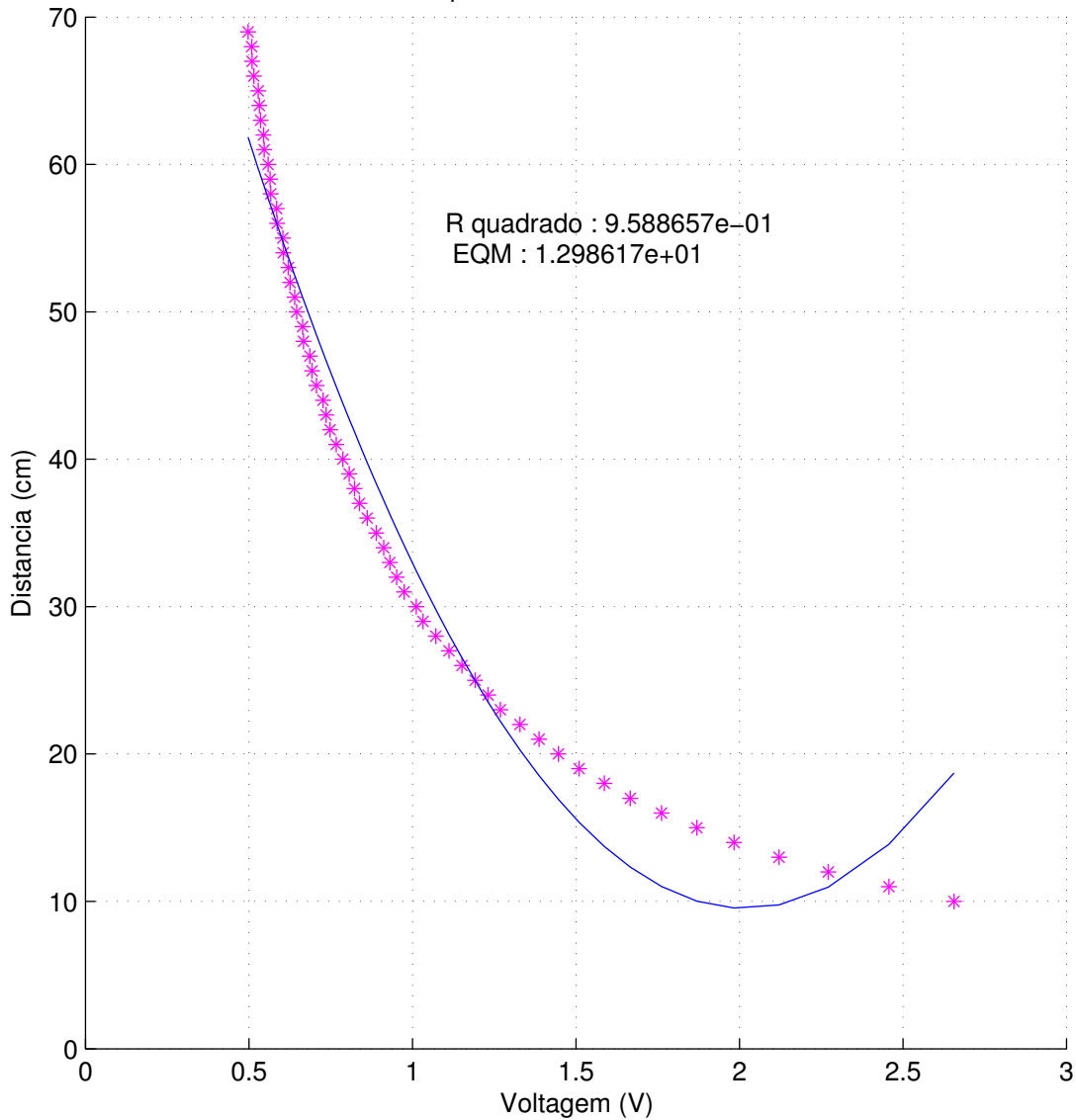
Polinomio ordem 2 para medidas de 1 em 1 cm com FANUC
