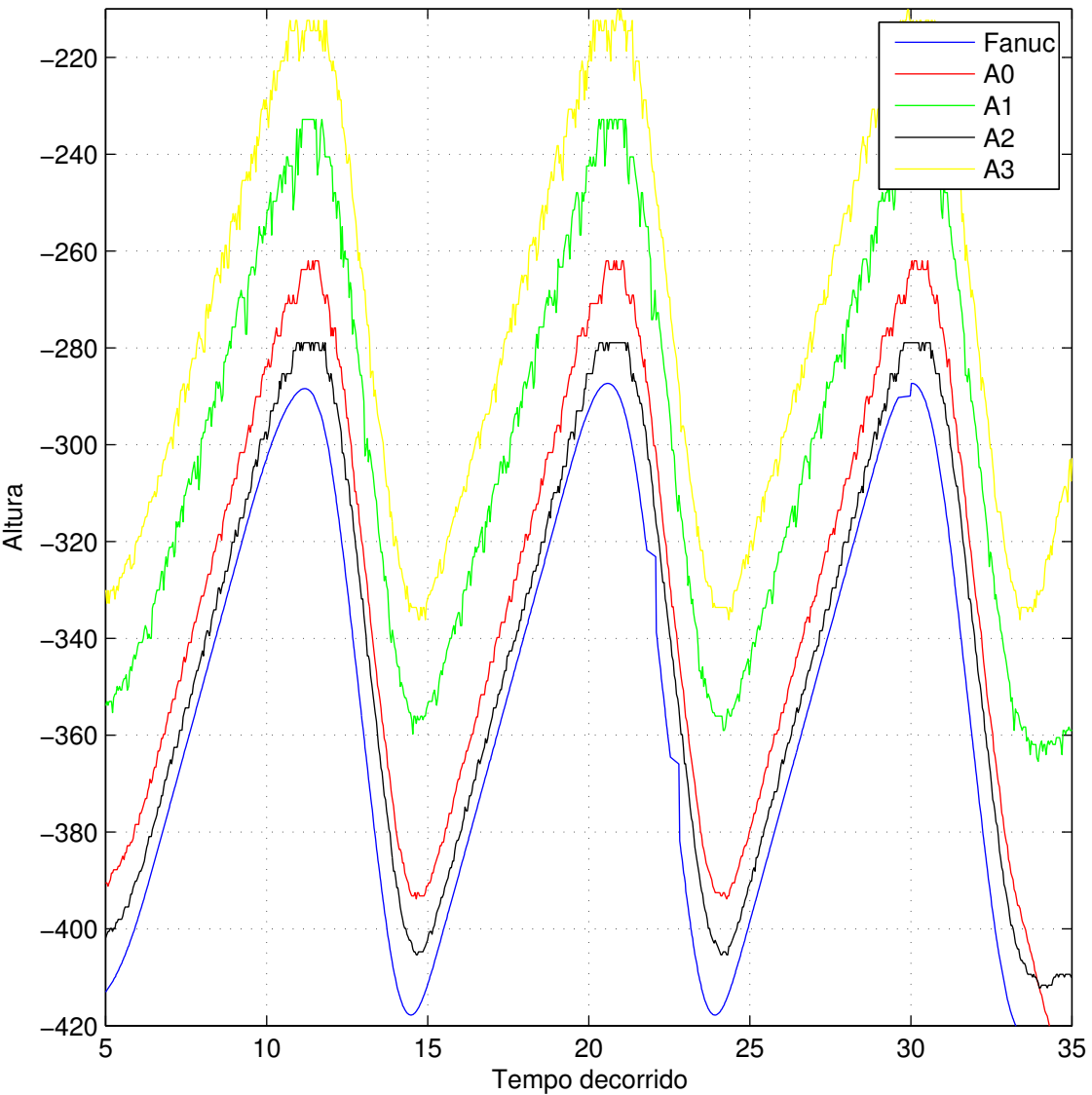
Altura lida do fanuc no seu referencial global e sensores.
