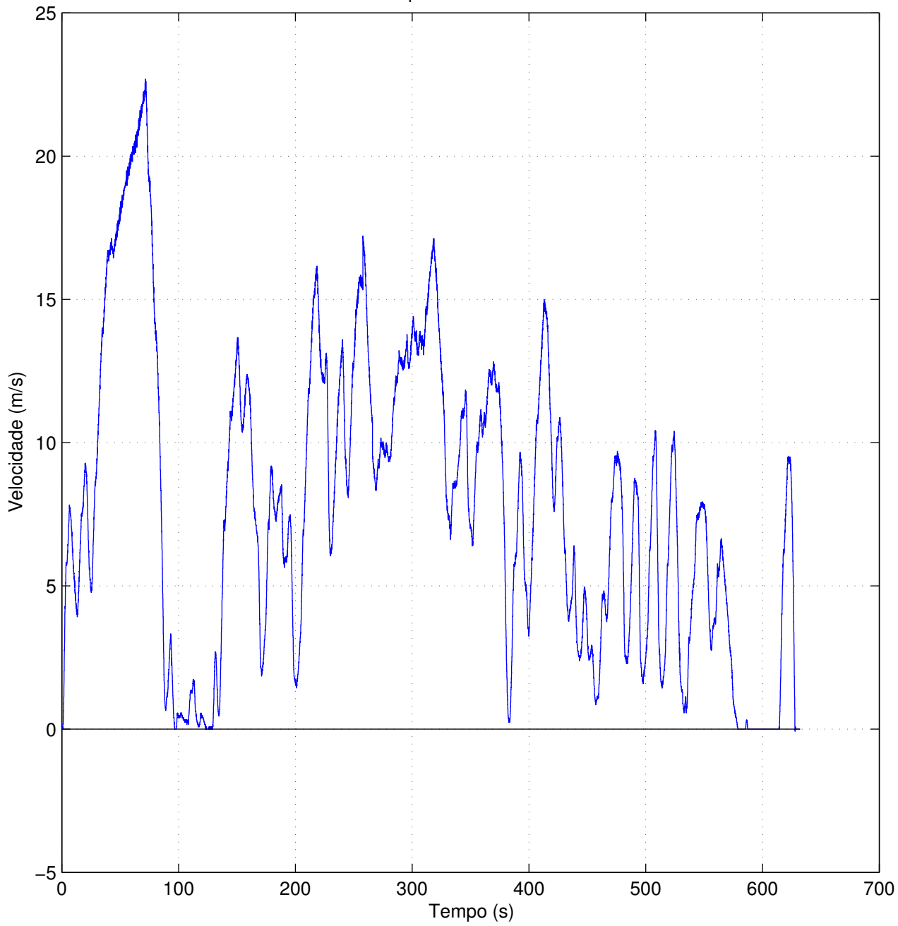
Dados obtidos para a velocidade do atlascar.
