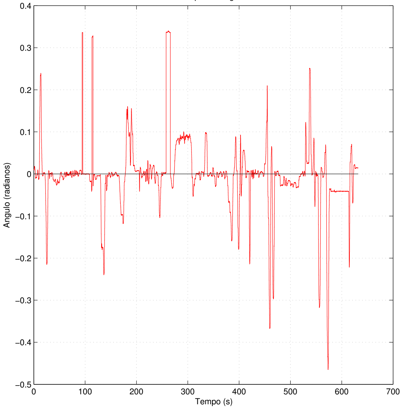
Dados obtidos para a angulo do volante.
