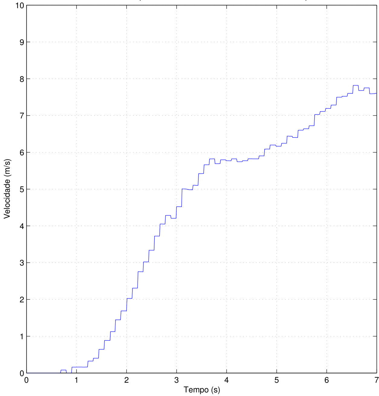
Dados obtidos para a velocidade do atlascar durante o arranque.
