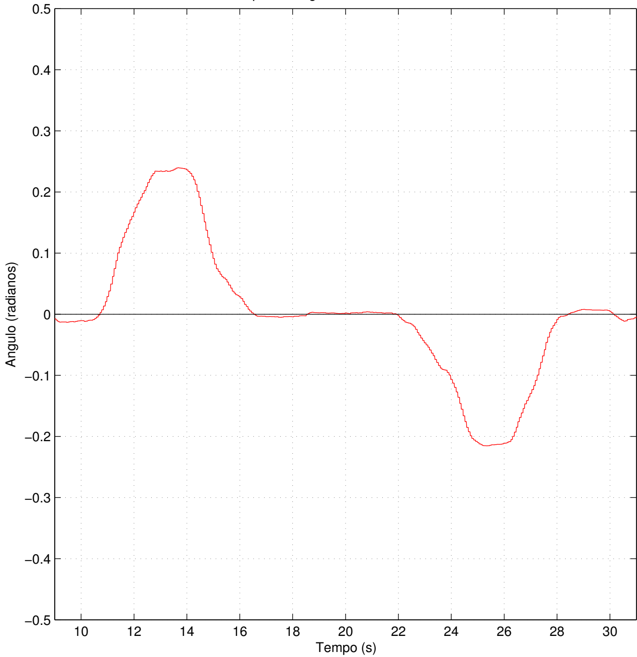
Dados obtidos para a angulo do volante durante duas curvas.
