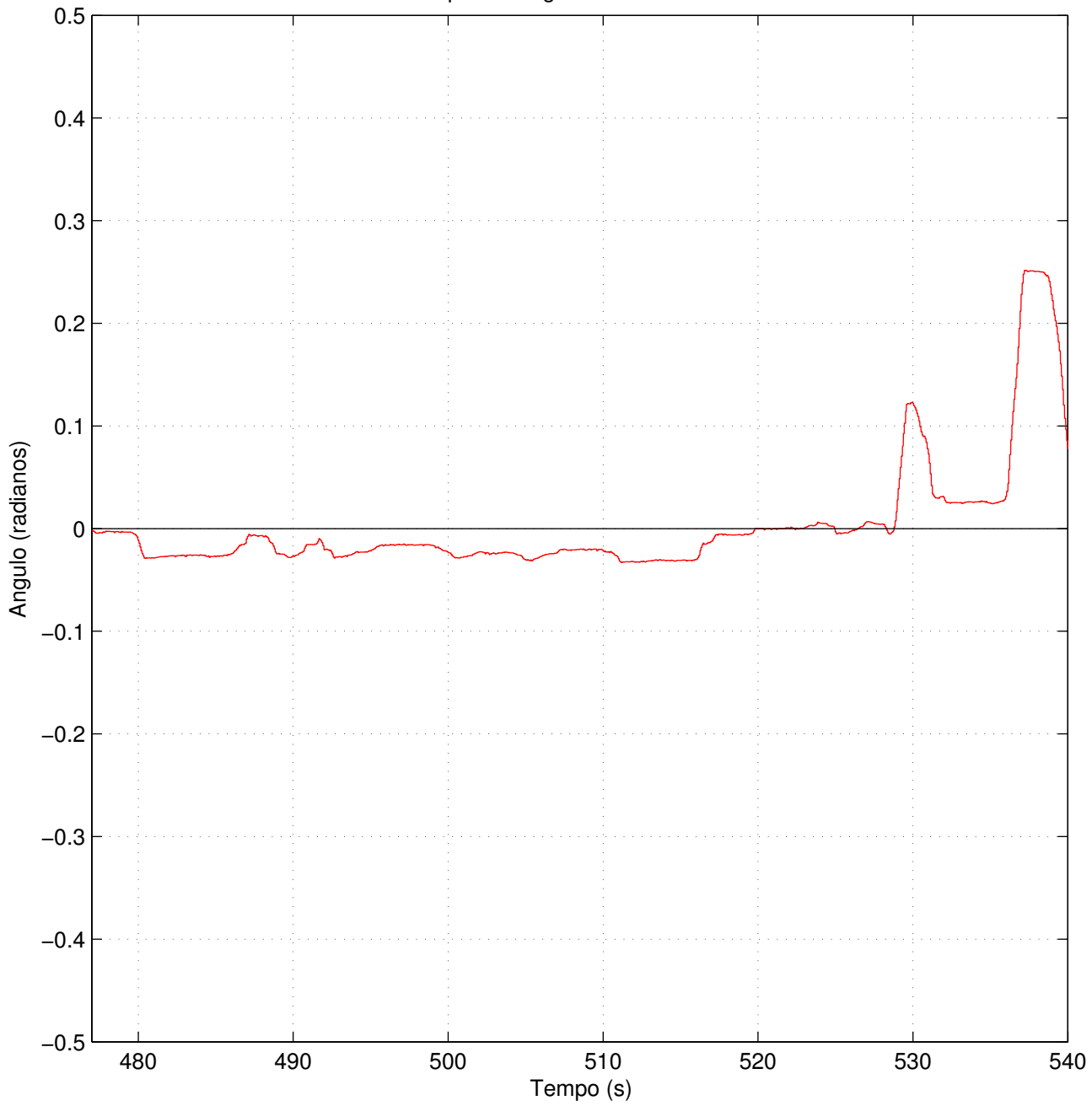
Dados obtidos para a angulo do volante durante lombas.
