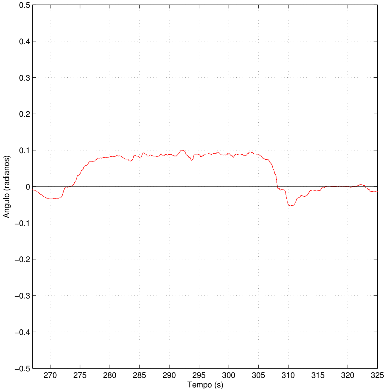
Dados obtidos para a angulo do volante numa rotunda.
