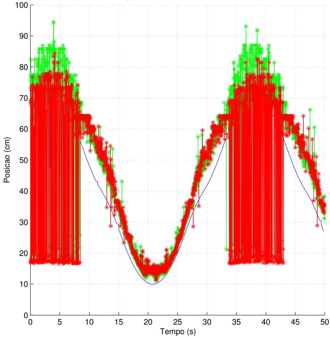
Fanuc movimento circular para simular seno e leitura do sensor nesse movimento
