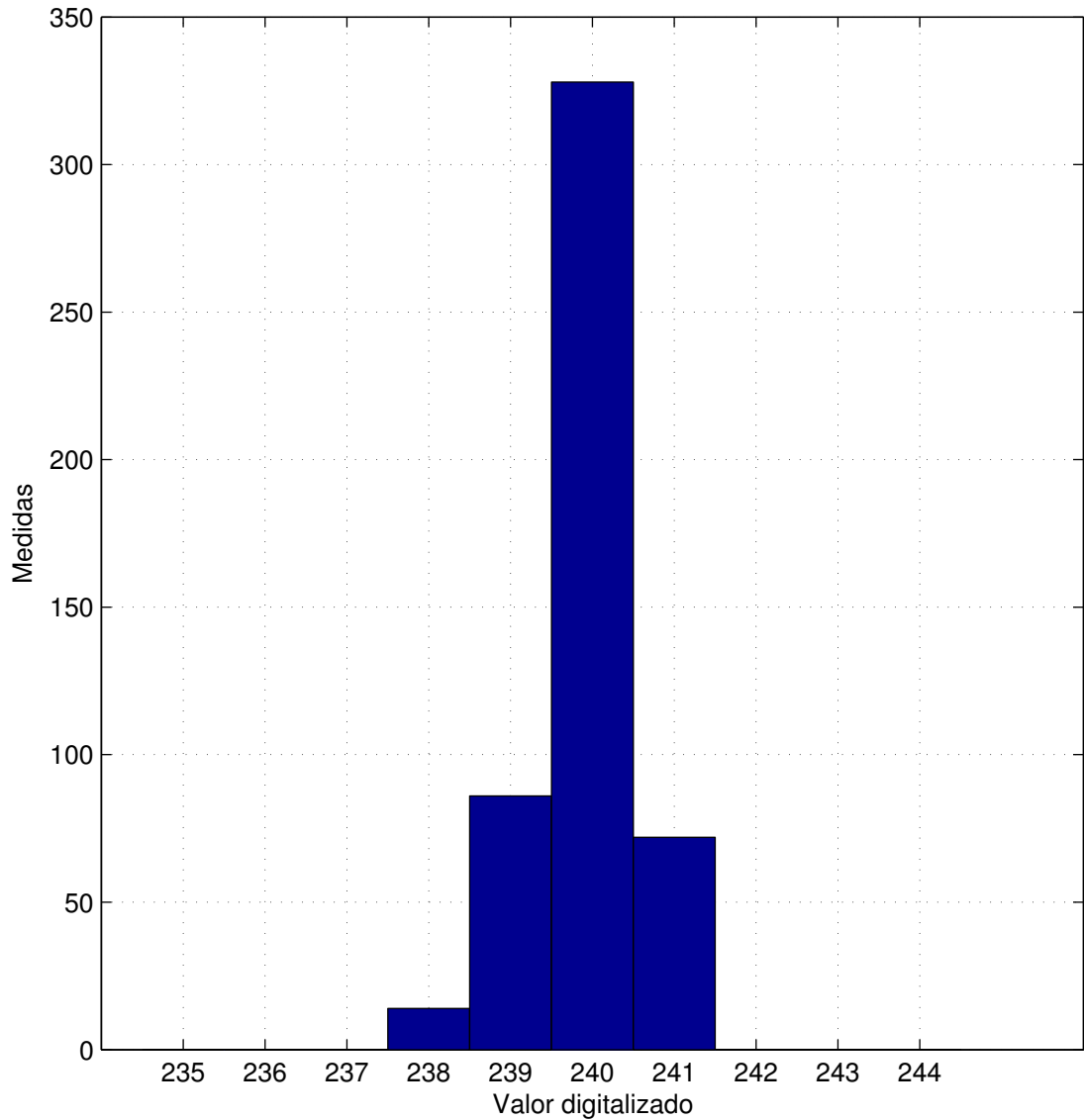
Teste de estabilidade do sensor em laboratório com filtro.
