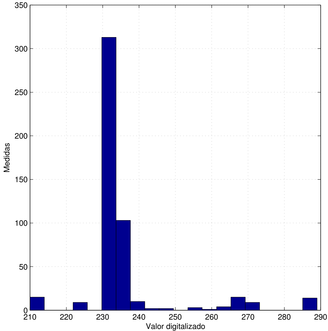
Teste de estabilidade do sensor em laboratório sem filtro.
