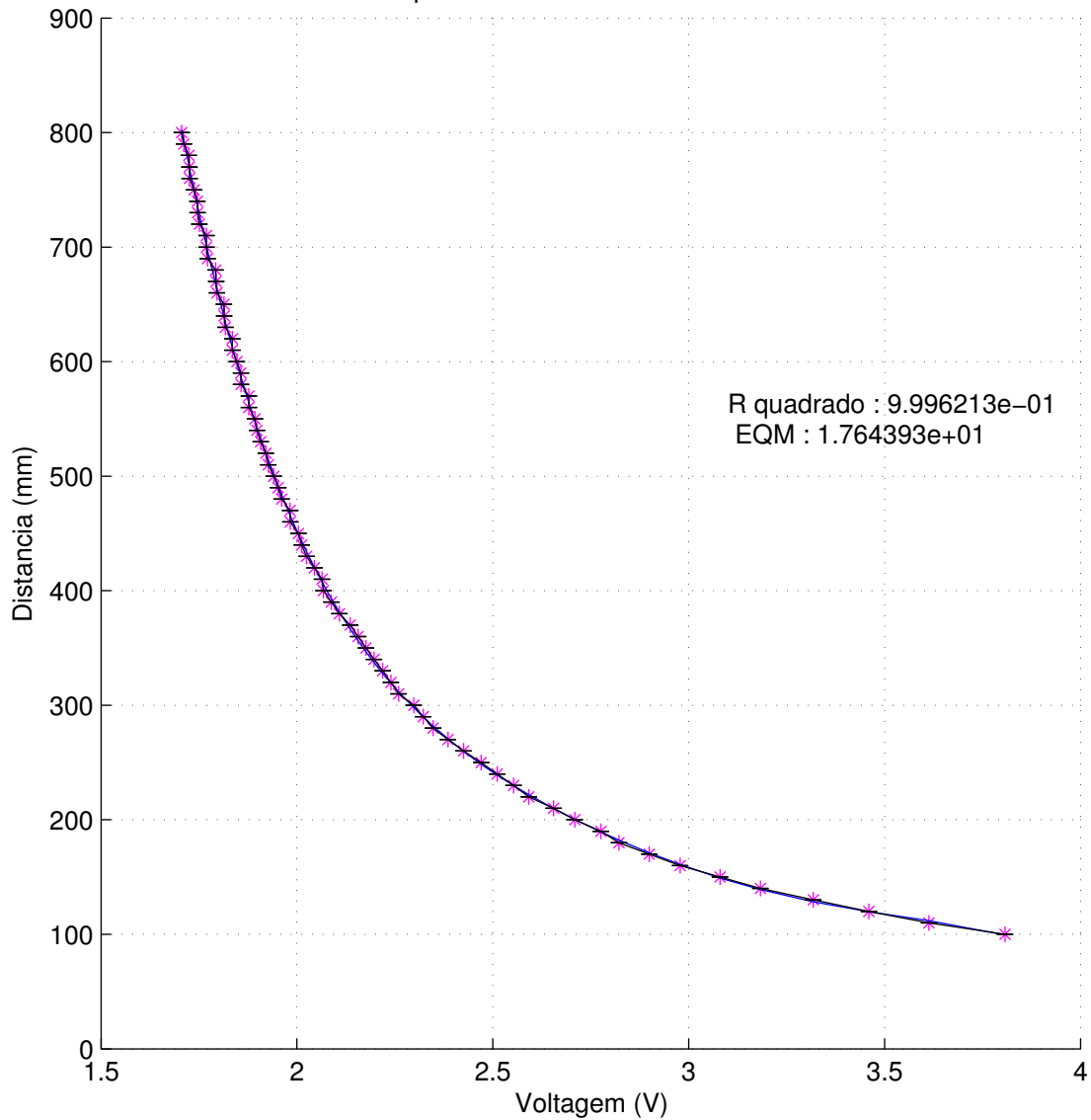
Polinomio ordem 6 para medidas de 10 em 10 mm com o robo Fanuc
