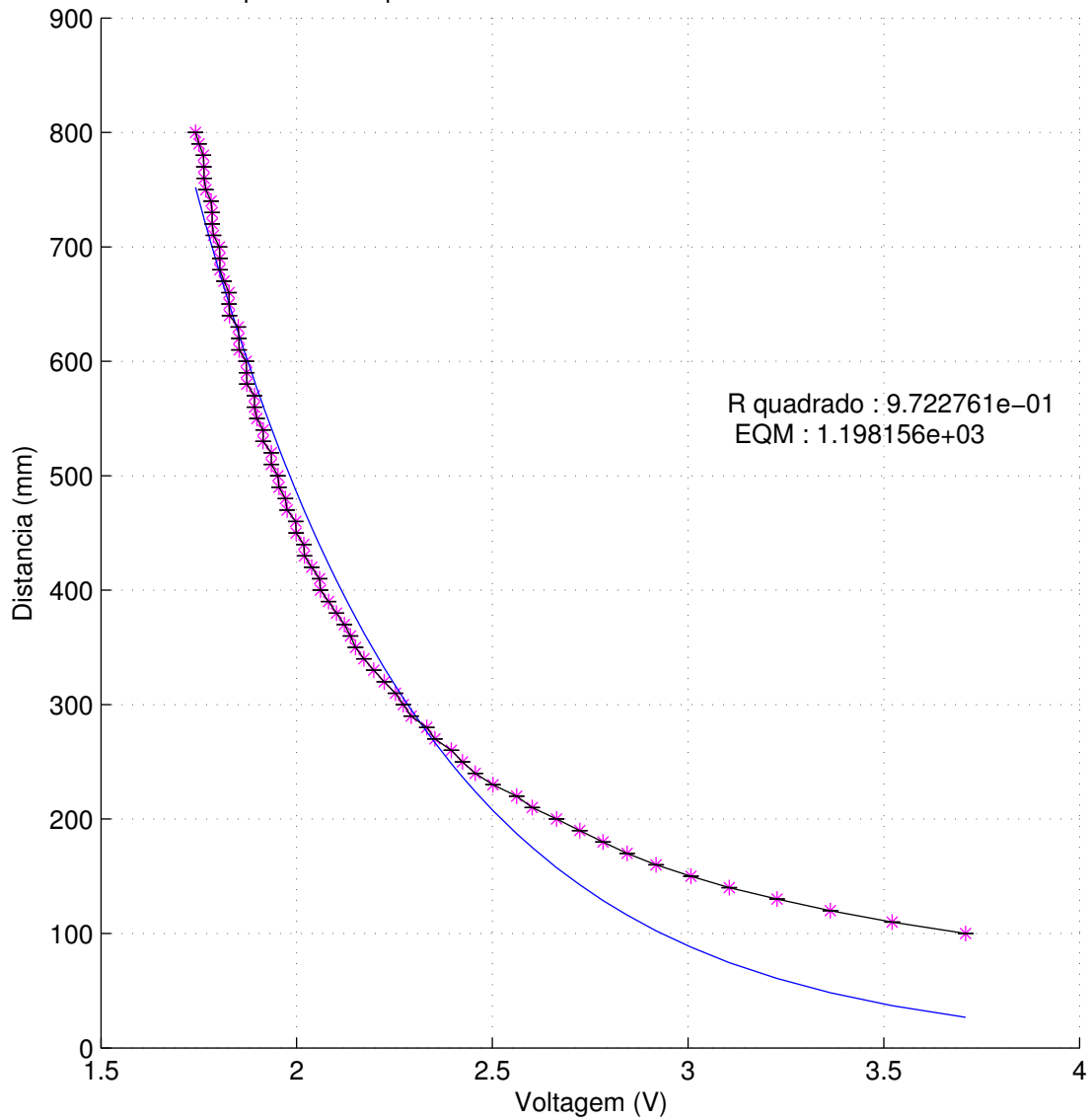
Exponencial 1 para medidas de 10 em 10 mm com o robo Fanuc
