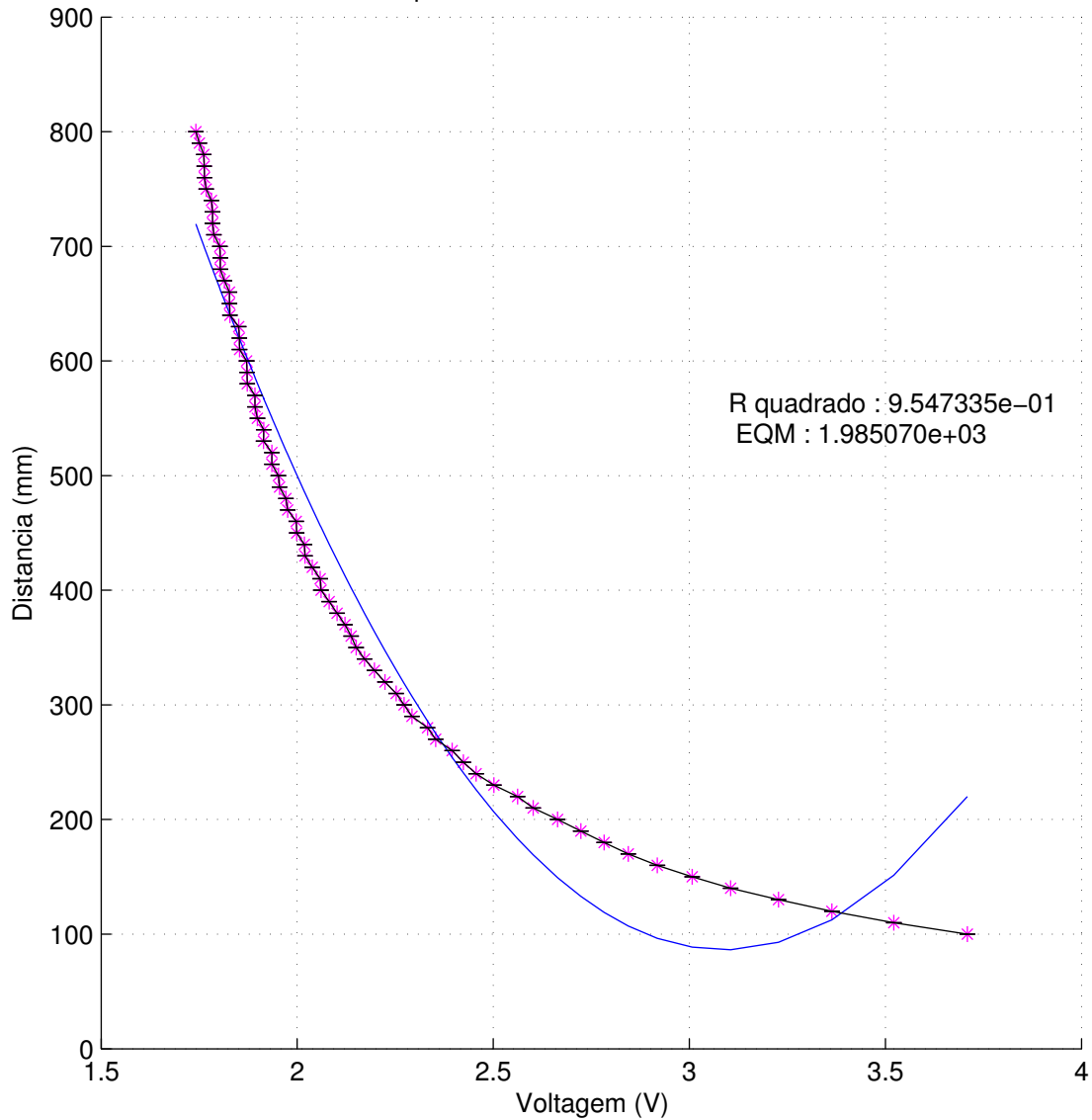
Polinomio ordem 2 para medidas de 10 em 10 mm com o robo Fanuc
