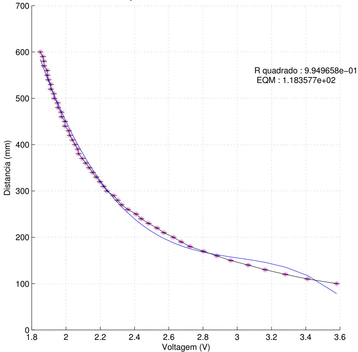
Polinomio ordem 3 para medidas de 10 em 10 mm com o robo Fanuc
