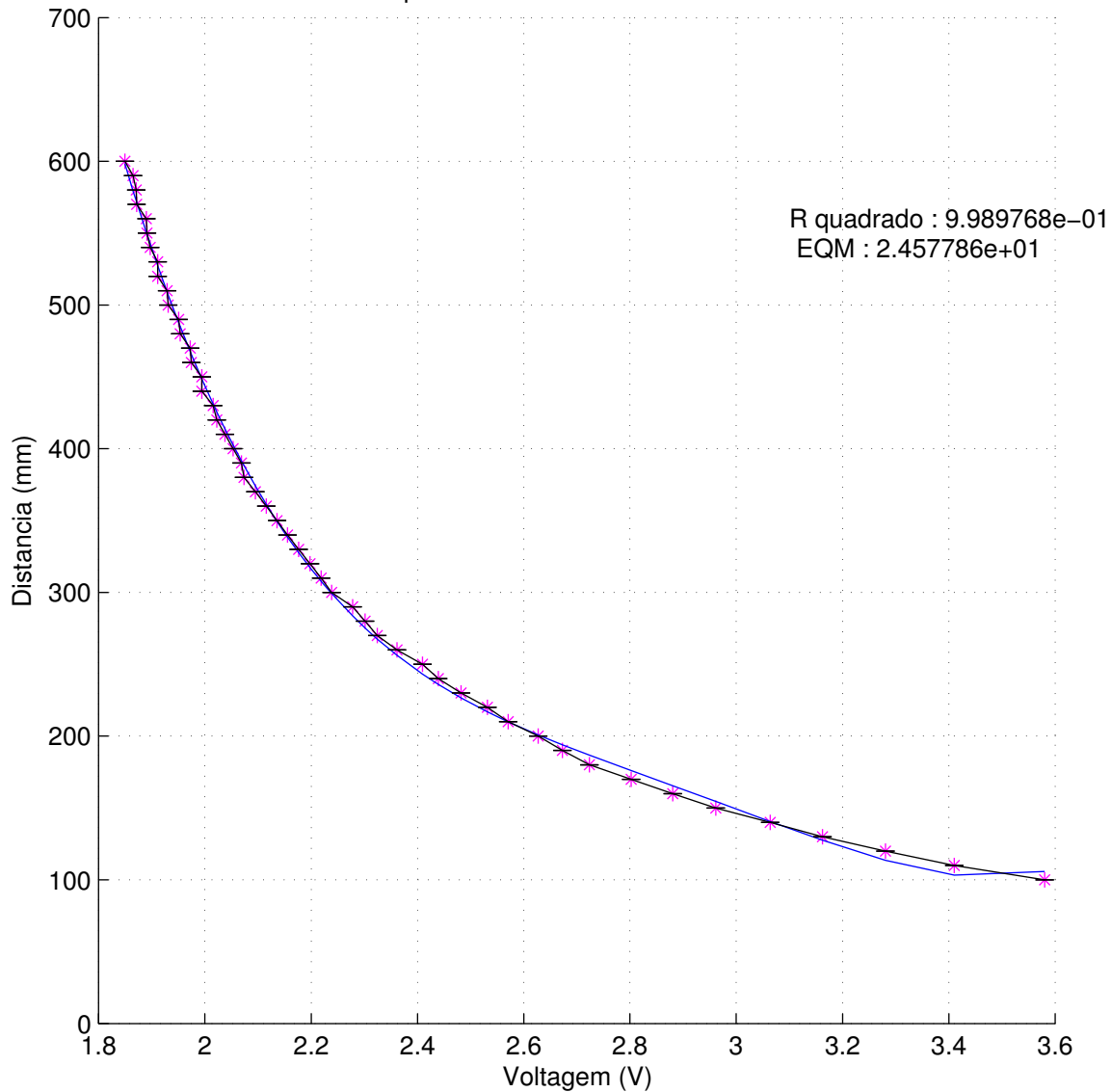
Polinomio ordem 4 para medidas de 10 em 10 mm com o robo Fanuc
