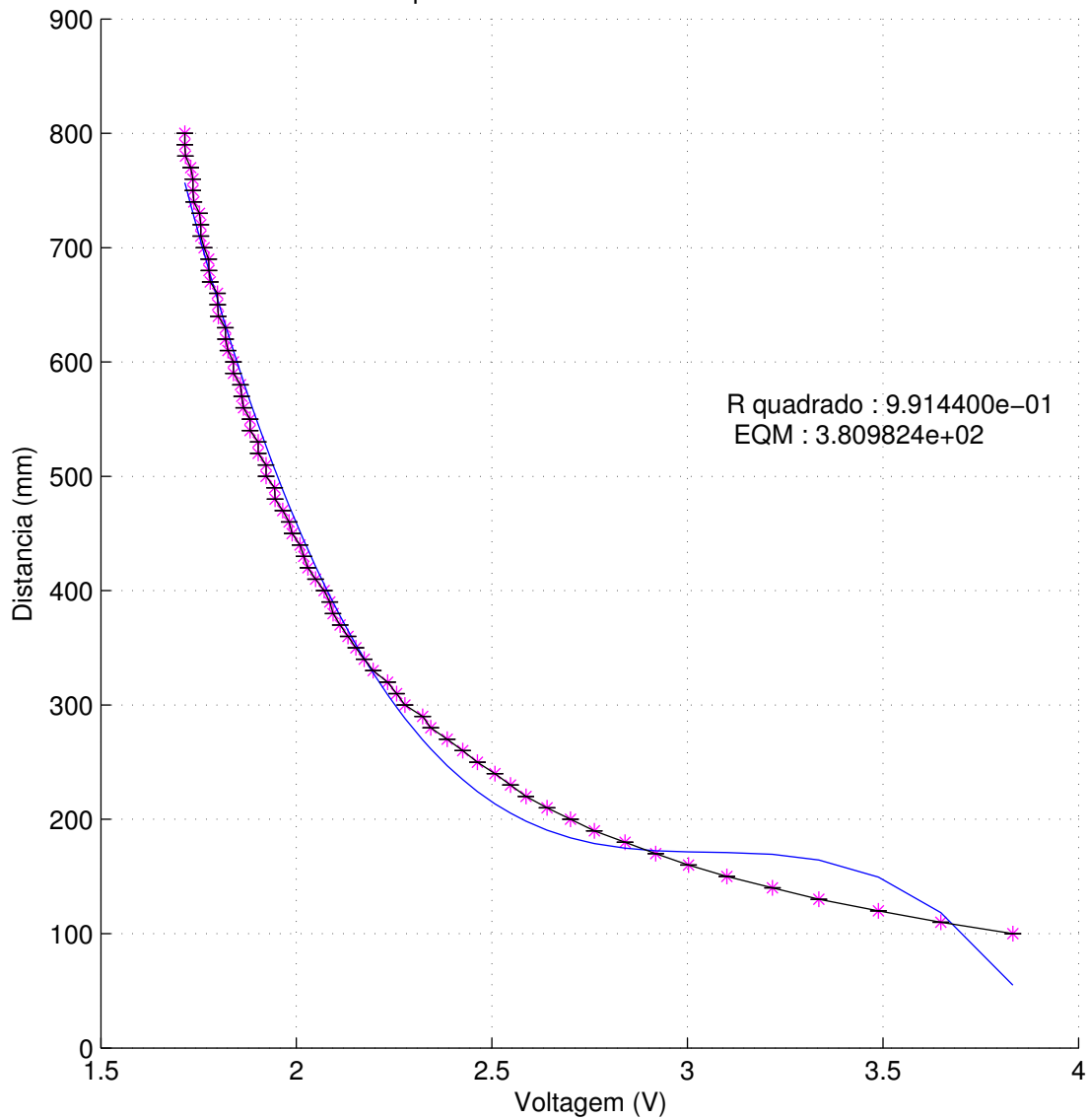
Polinômio ordem 3 para medidas de 10 em 10 mm com o robo Fanuc
