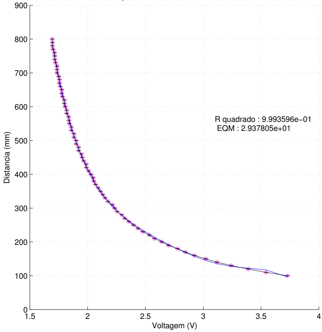
Polinomio ordem 5 para medidas de 10 em 10 mm com o robo Fanuc
