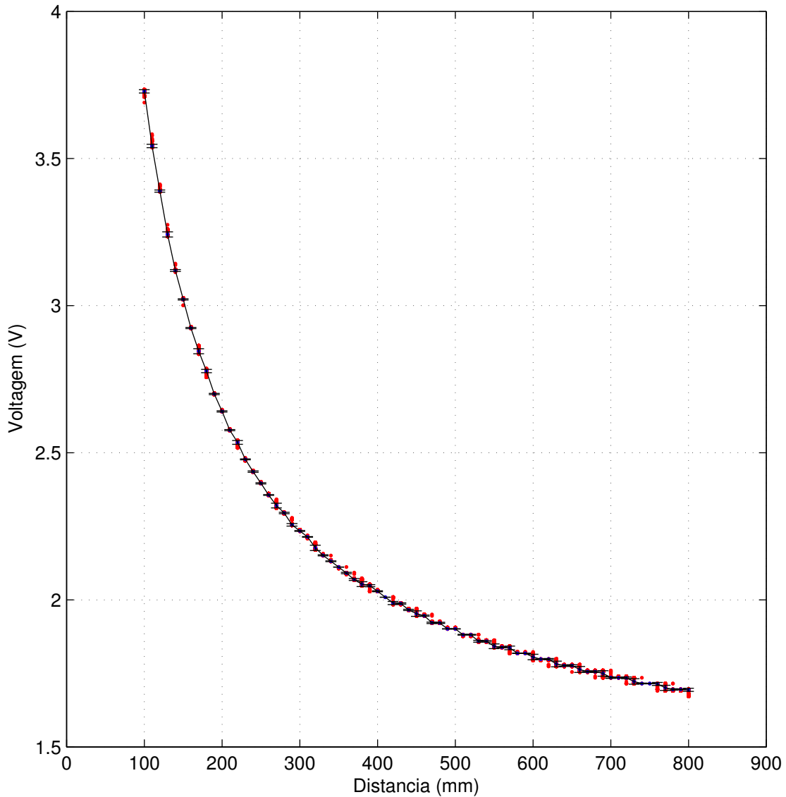
Valores obtidos de 10 em 10 mm com o robo Fanuc
