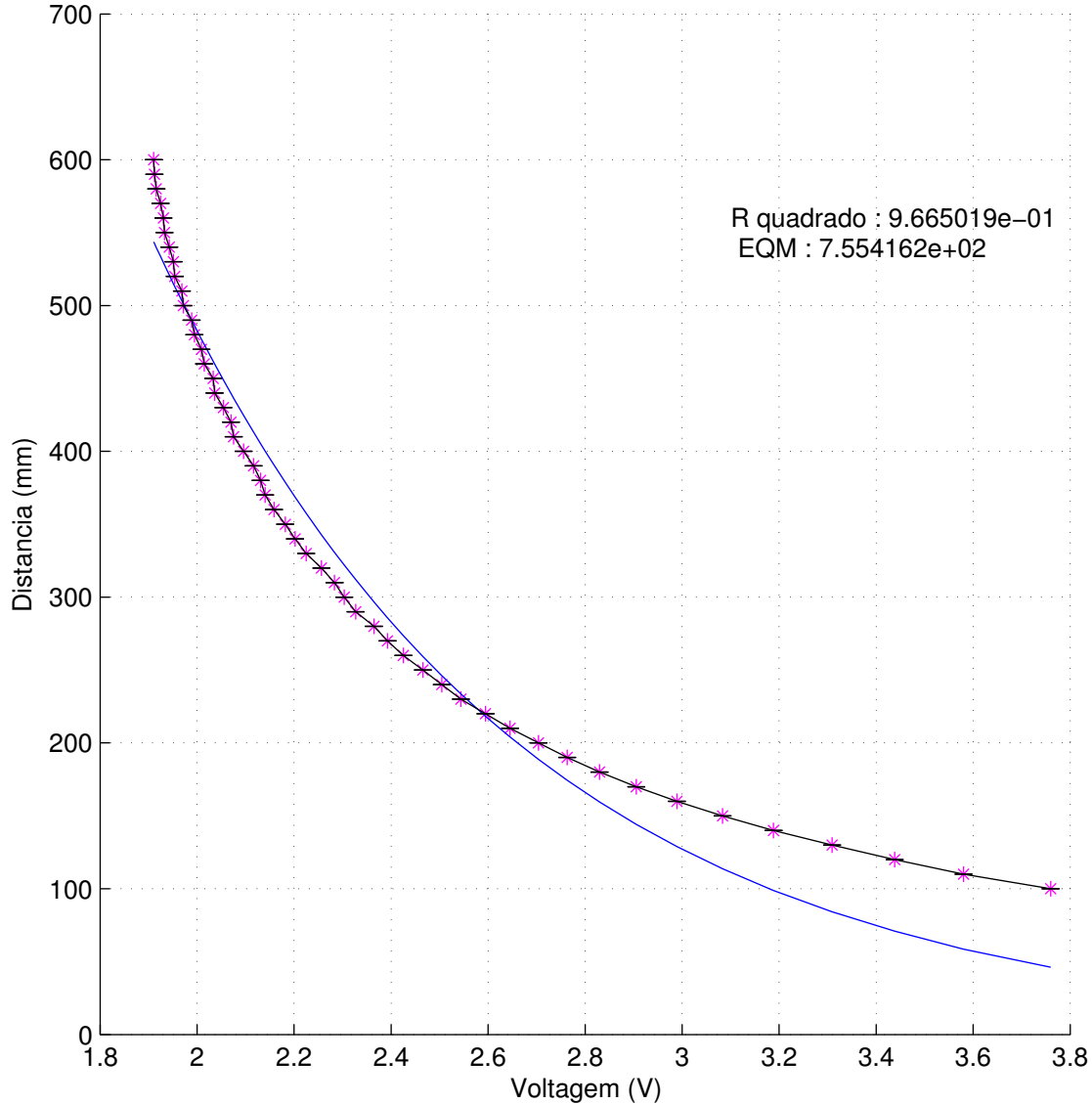
Exponencial 1 para medidas de 10 em 10 mm com o robo Fanuc
