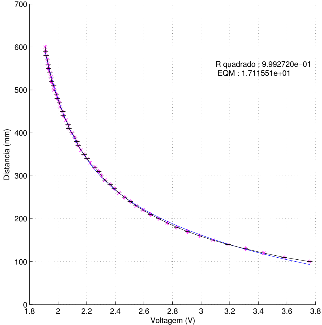
Exponencial 2 para medidas de 10 em 10 mm com o robo Fanuc
