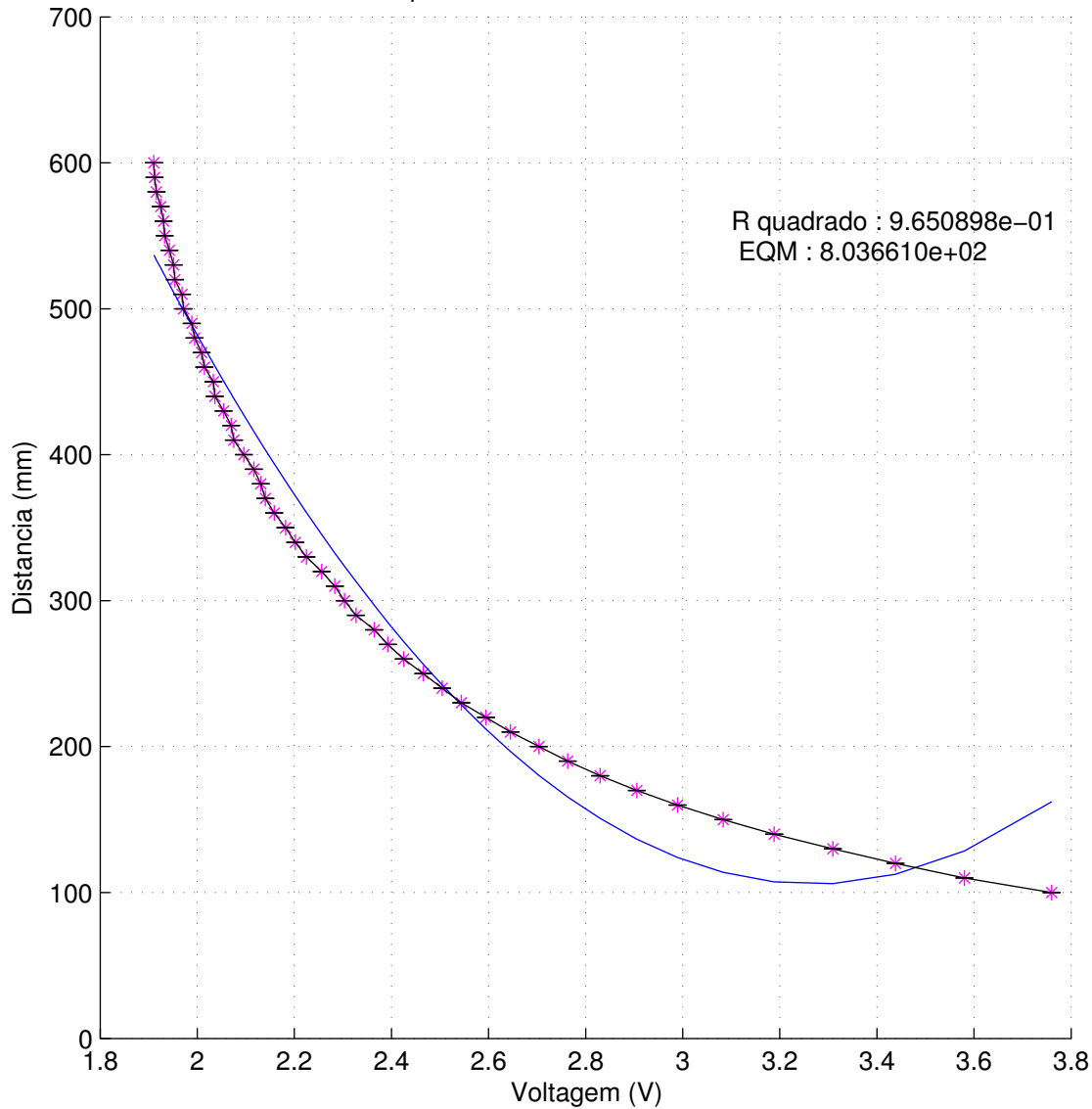
Polinômio ordem 2 para medidas de 10 em 10 mm com o robo Fanuc
