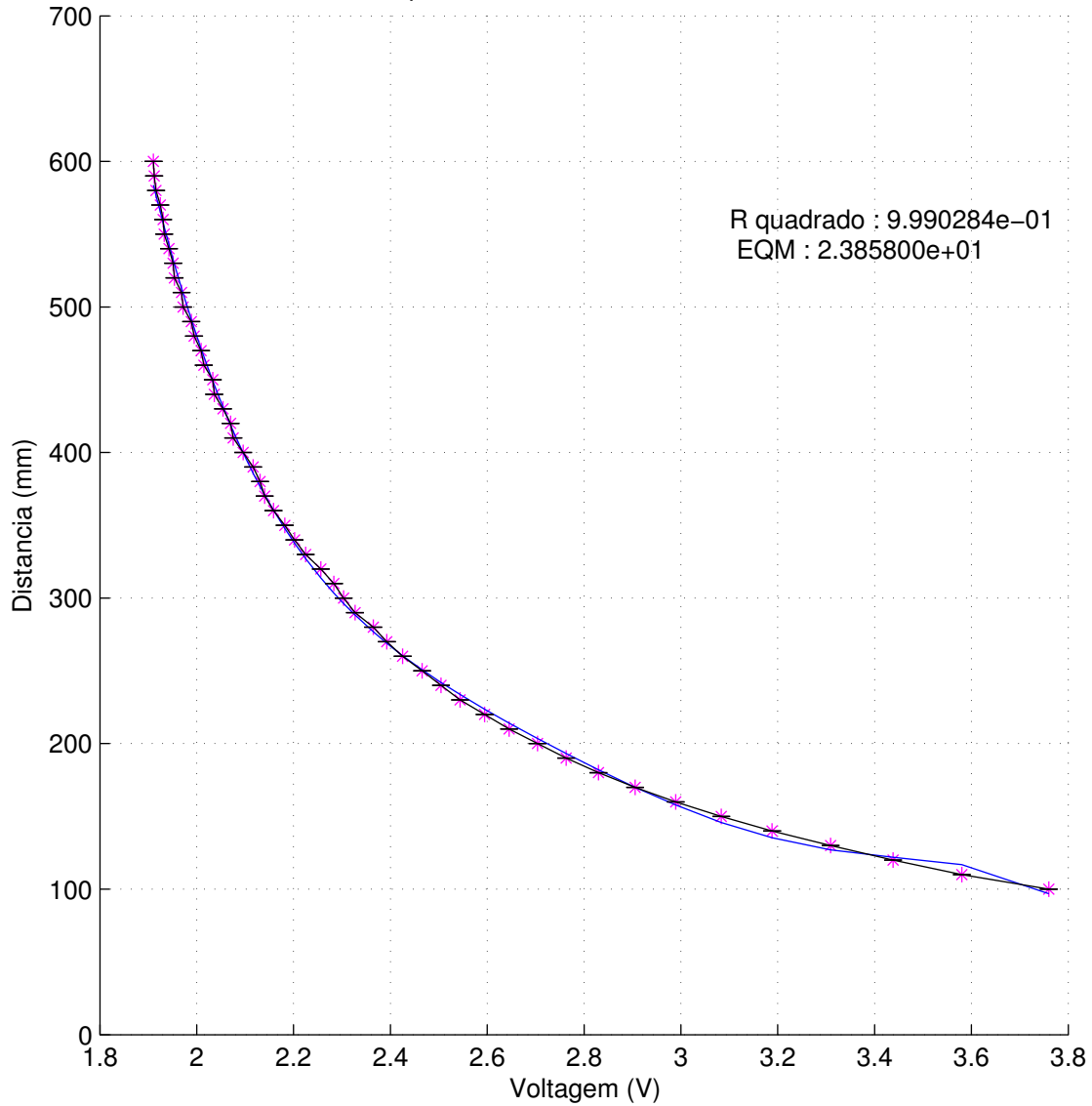
Polinomio ordem 5 para medidas de 10 em 10 mm com o robo Fanuc
