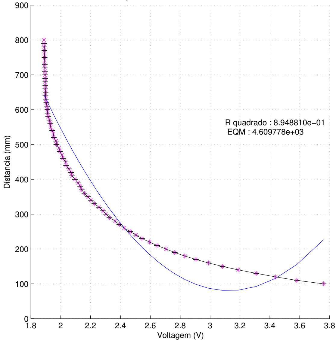
Polinomio ordem 2 para medidas de 10 em 10 mm com o robo Fanuc
