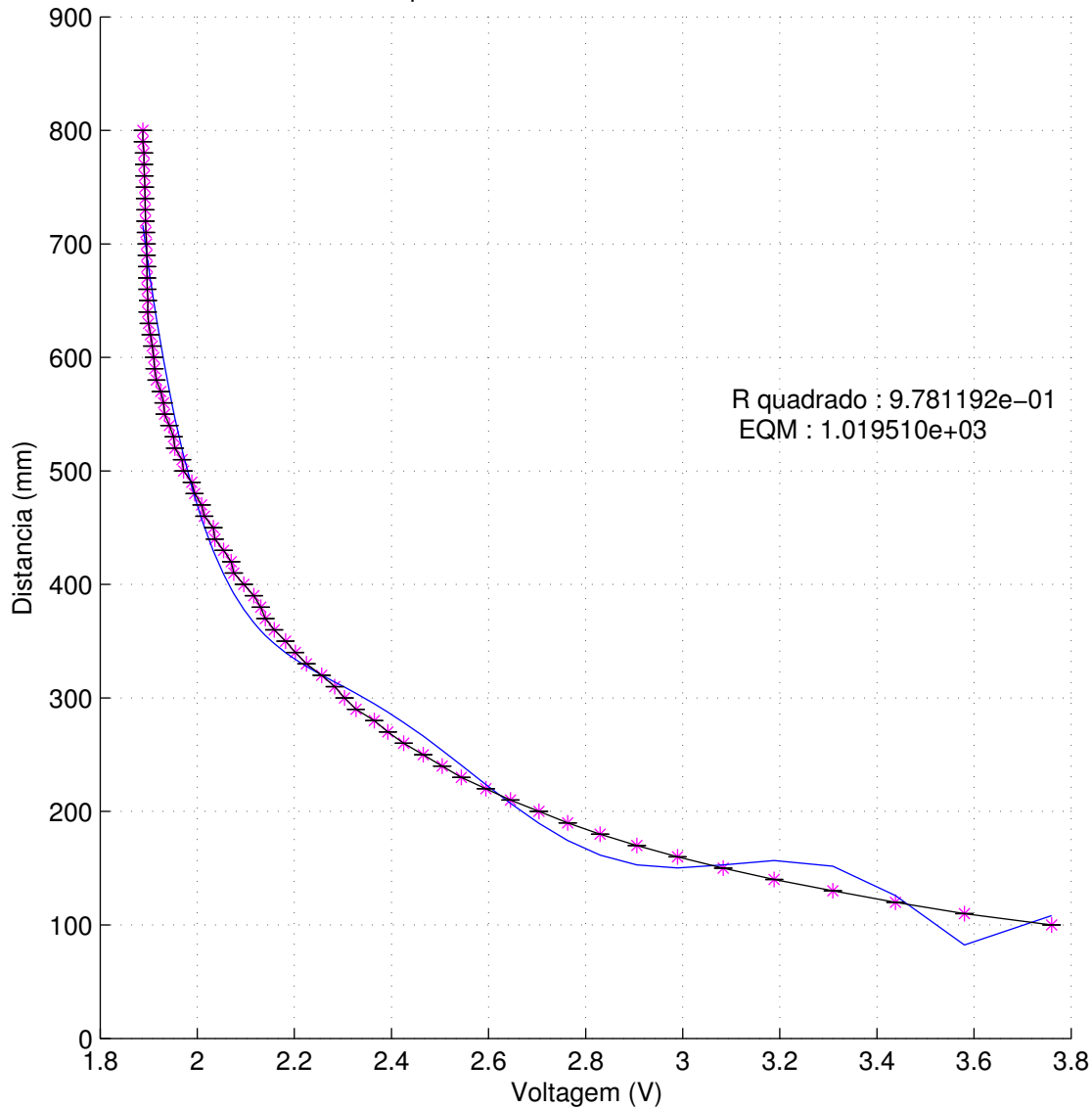
Polinomio ordem 6 para medidas de 10 em 10 mm com o robo Fanuc
