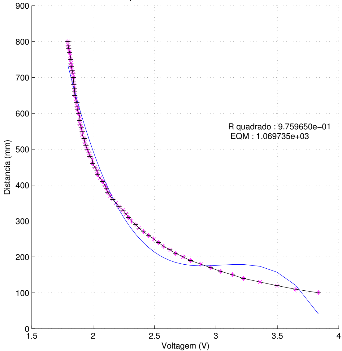
Polinomio ordem 3 para medidas de 10 em 10 mm com o robo Fanuc
