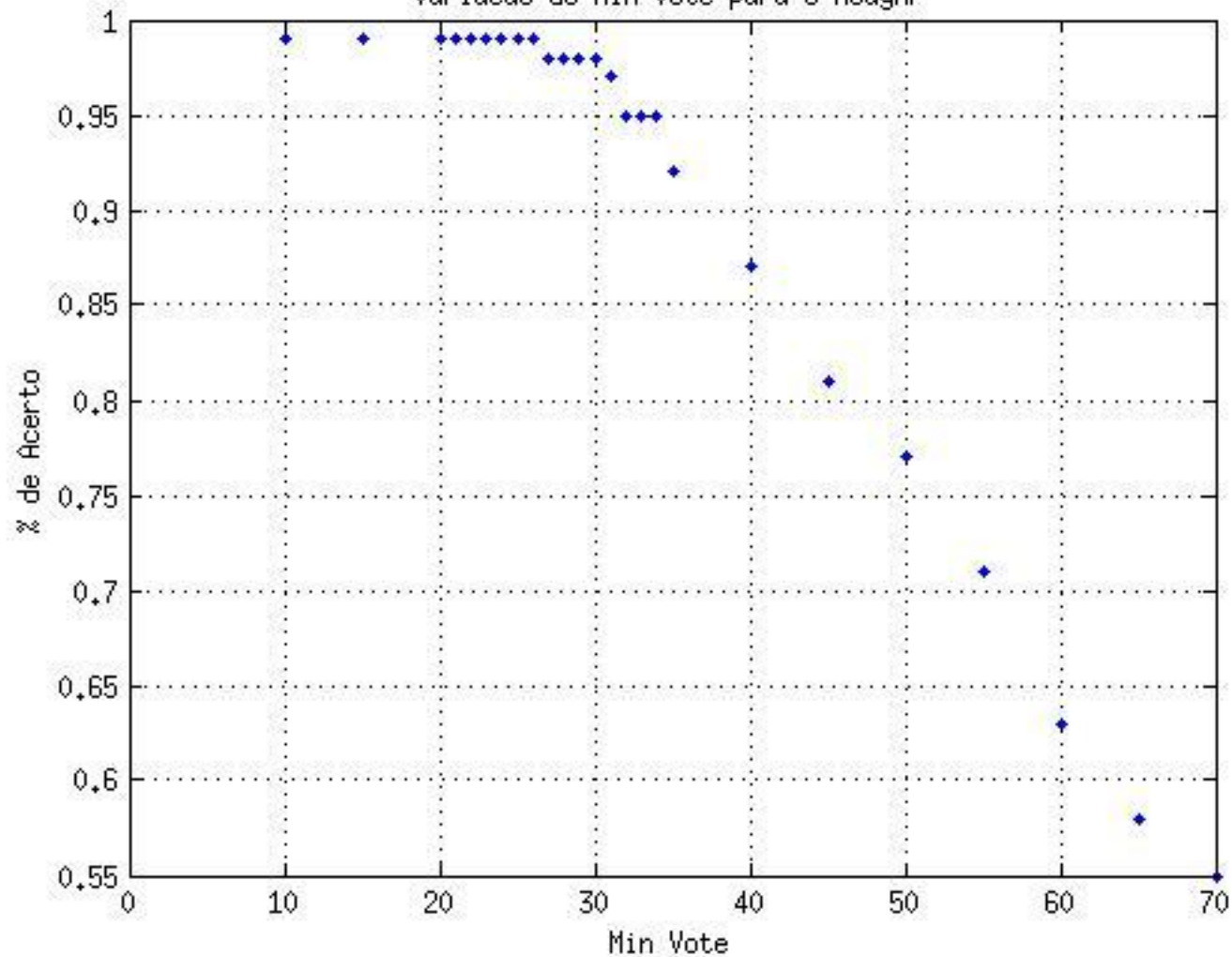
Variacao do Min Vote para o HoughP
